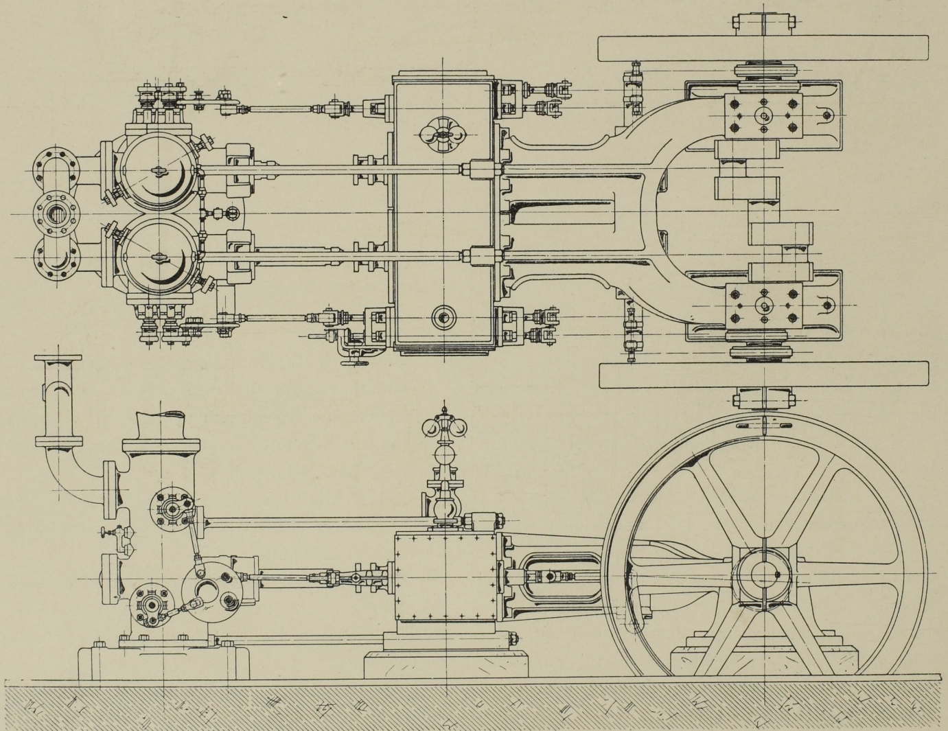
Abb. 55. Seitenansicht und Grundriss der Maschine. Massst. 1:36.
