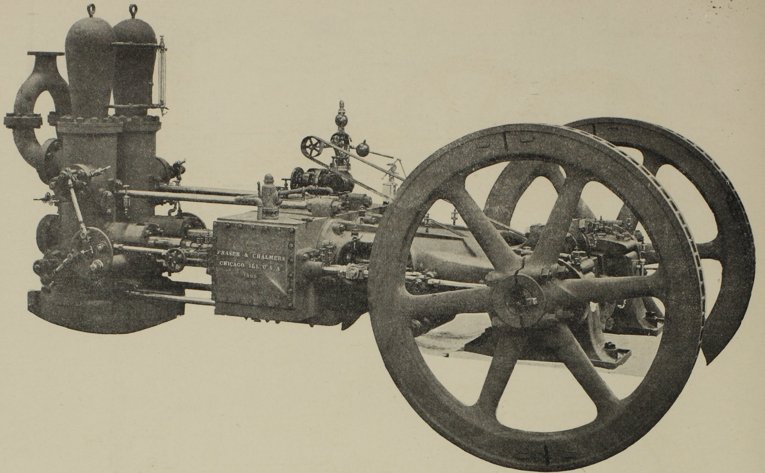
Abb 54. Gesamtbild der Maschine.
