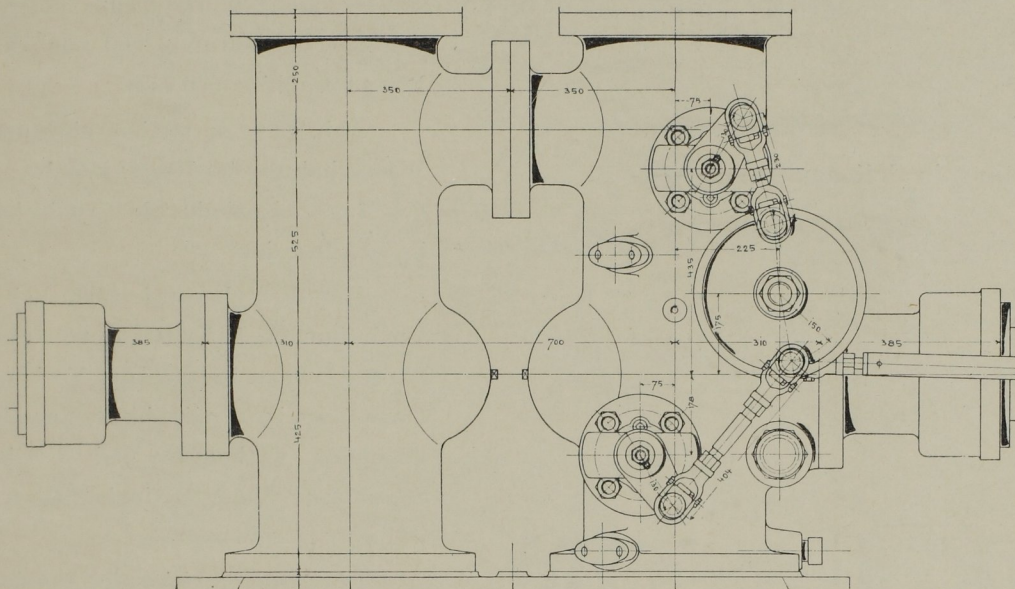
Abb. 29. Seitenansicht und Pumpensteuerung. Massst. 1:5.
