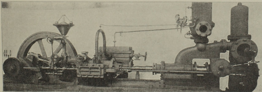
Abb. 30. Einachsige Wasserhaltungsmaschine, gebaut von Breitfeld, Danek & Co. in Prag.
