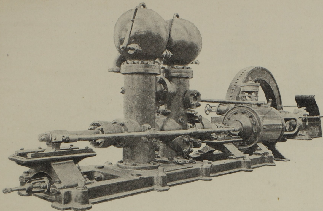
Abb. 28. Wasserhaltung des Karl-Schachtes in Karwin bei Mähr.-Ostrau.
