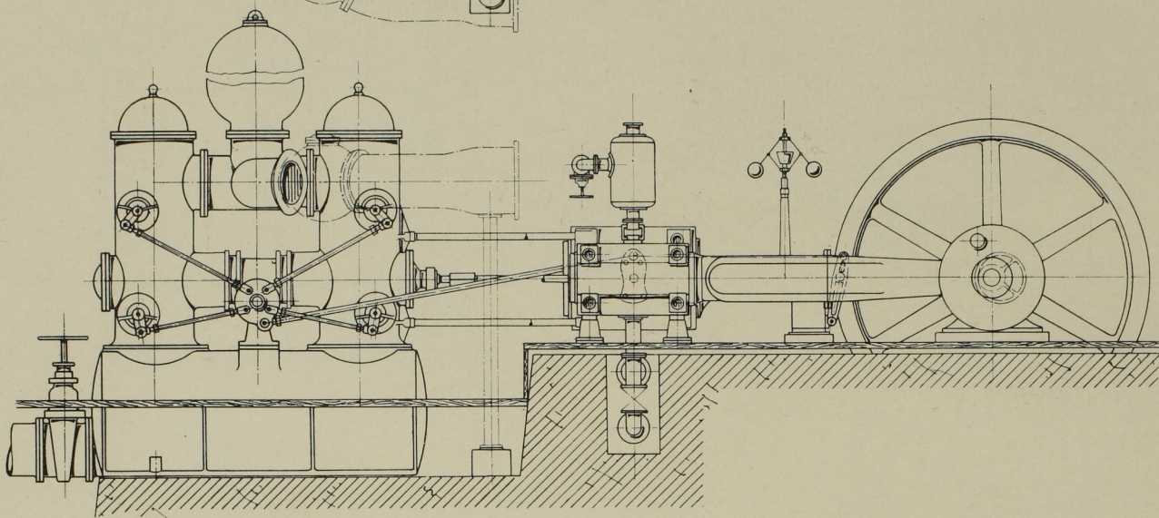
Abb. 33. Seitenansicht. Masst. 1 : 75.
