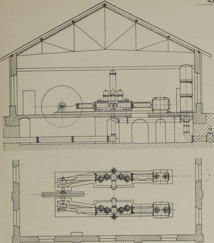
Abb. 95. Gesamtanordnung. Massst. 1:150. Wasserwerk Stuttgart-Bergstrasse.
