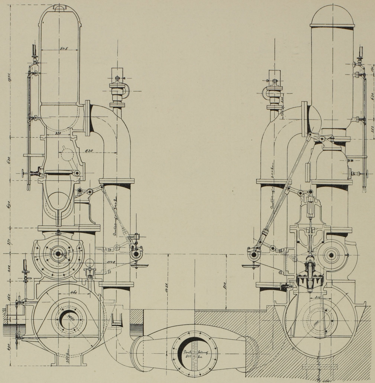
Abb. 93. Querschnitt der Druckpumpen und Pumpensteuerung. Masst. 1:30.
