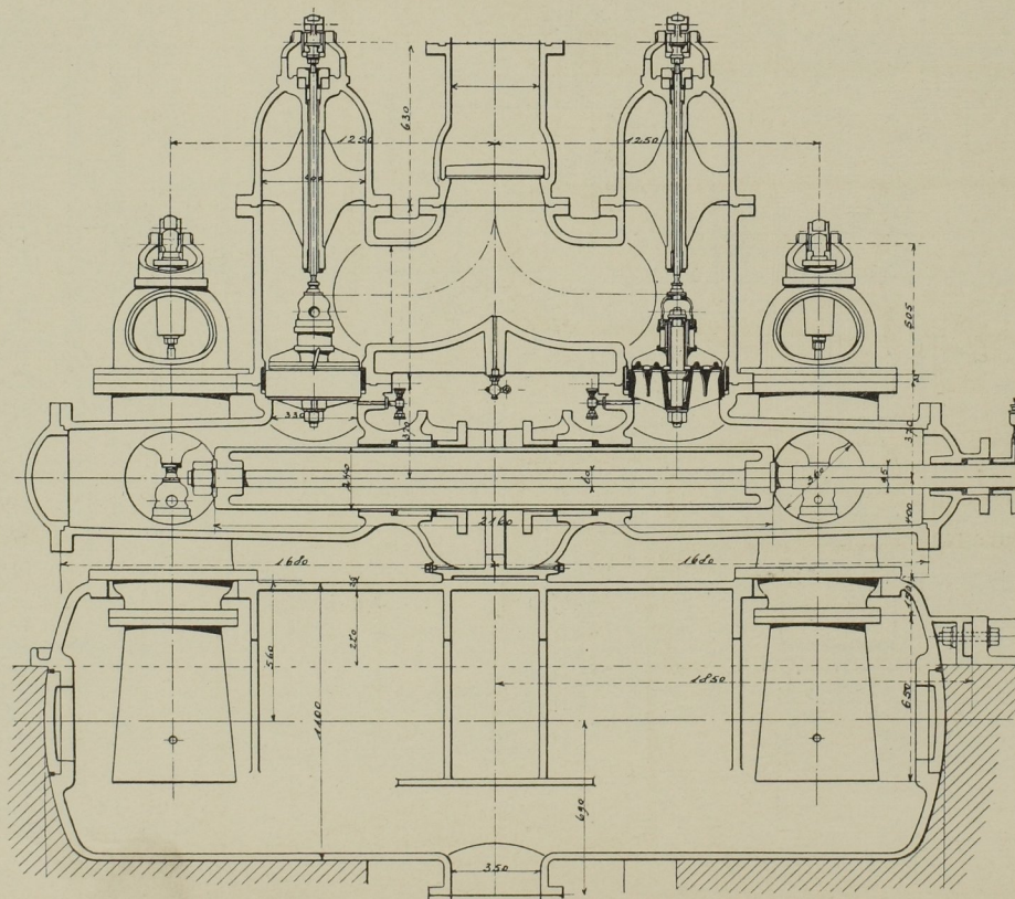
Abb. 94. Längsschnitt durch die Druckpumpe. Masst. 1:30. Pumpmaschine des Wasserwerks Witten a. Ruhr.
