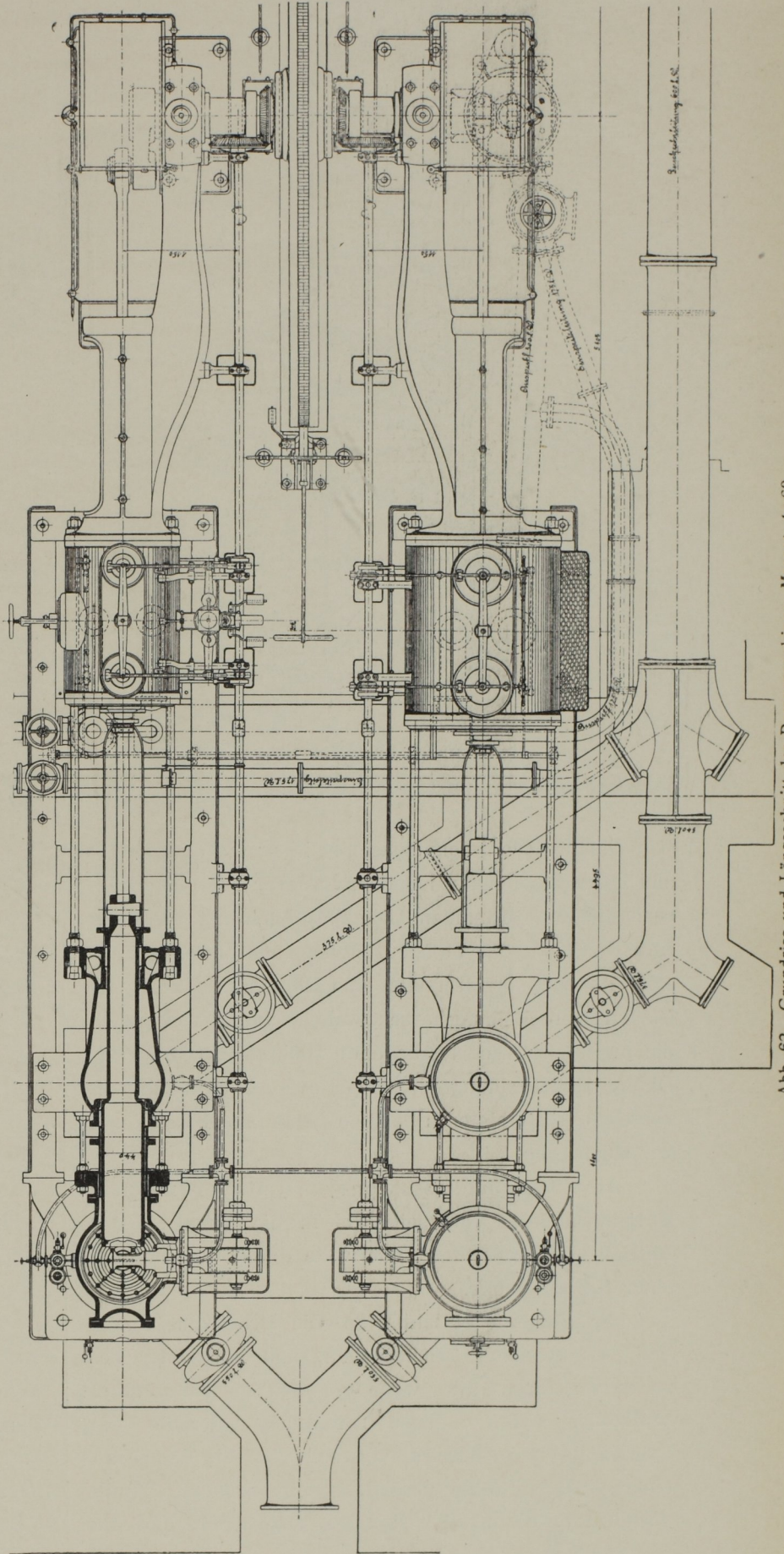
Abb. 62. Grundriss und Längsschnitt der Pumpmaschine. Massst. 1:60.
