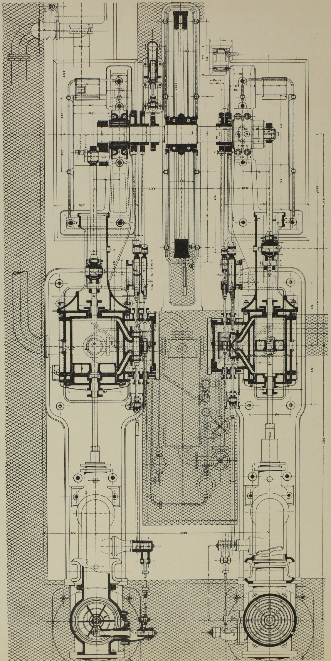
Abb. 8. Grundriss und Längsschnitt der Pumpmaschine. Massst. 1:30.
