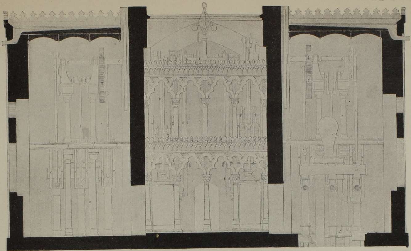
Abb. 2 Vorderansicht der Maschinen und Pumpen Masst. 1 : 90.
