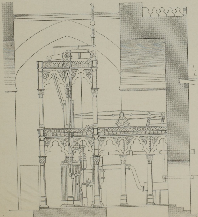
Abb. 4. Seitenansicht der Maschinen. Masst. 1 : 90.
