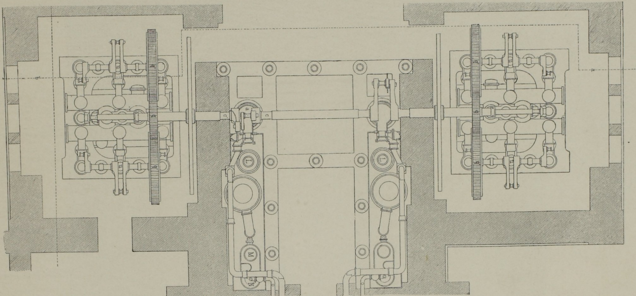
Abb. 3. Grundriss der Maschinen und Pumpen. Masst. 1 : 90.
