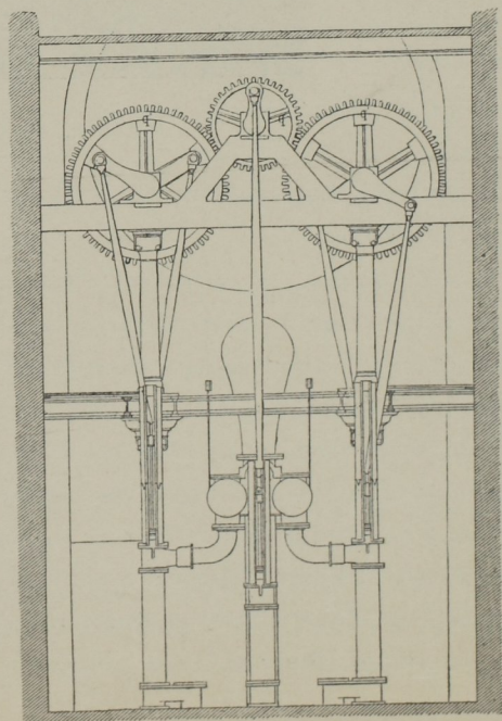
Abb. 5. Seitenansicht der Pumpen. Masst. 1 : 90.
