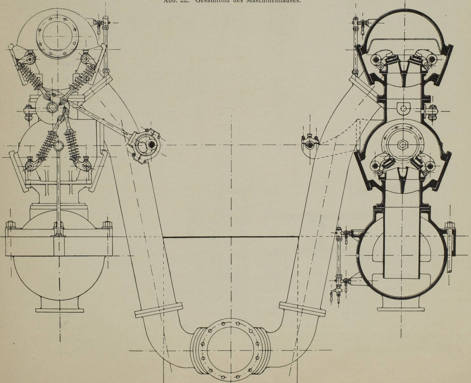
Abb. 23. Seitenansicht und Querschnitt der Druckpumpen. Massst. 1:20. Pumpenanlage der städtischen Kanalisation in Braunschweig.
