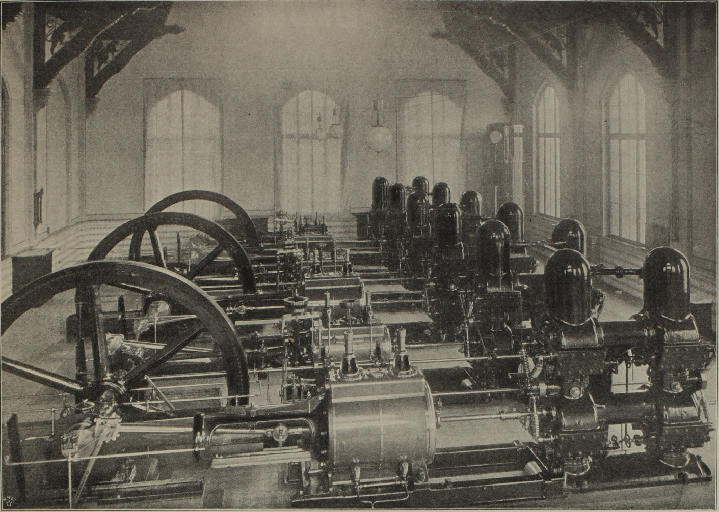
Abb. 22. Gesamtbild des Maschinenhauses.
