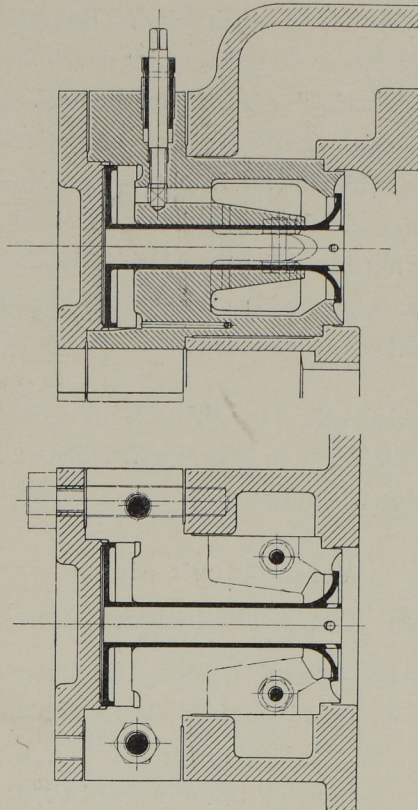
Abb. 8. Rückläufige Druckventile.
