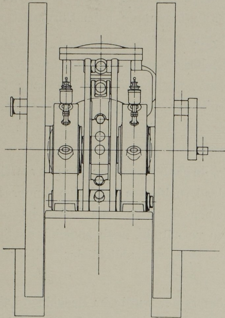
Abb. 7. Rückansicht. Masst. 1:15.
