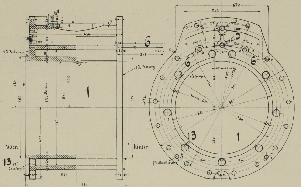
Abb. 24. Kompressor-Cylinder. Massst. 1:15.
