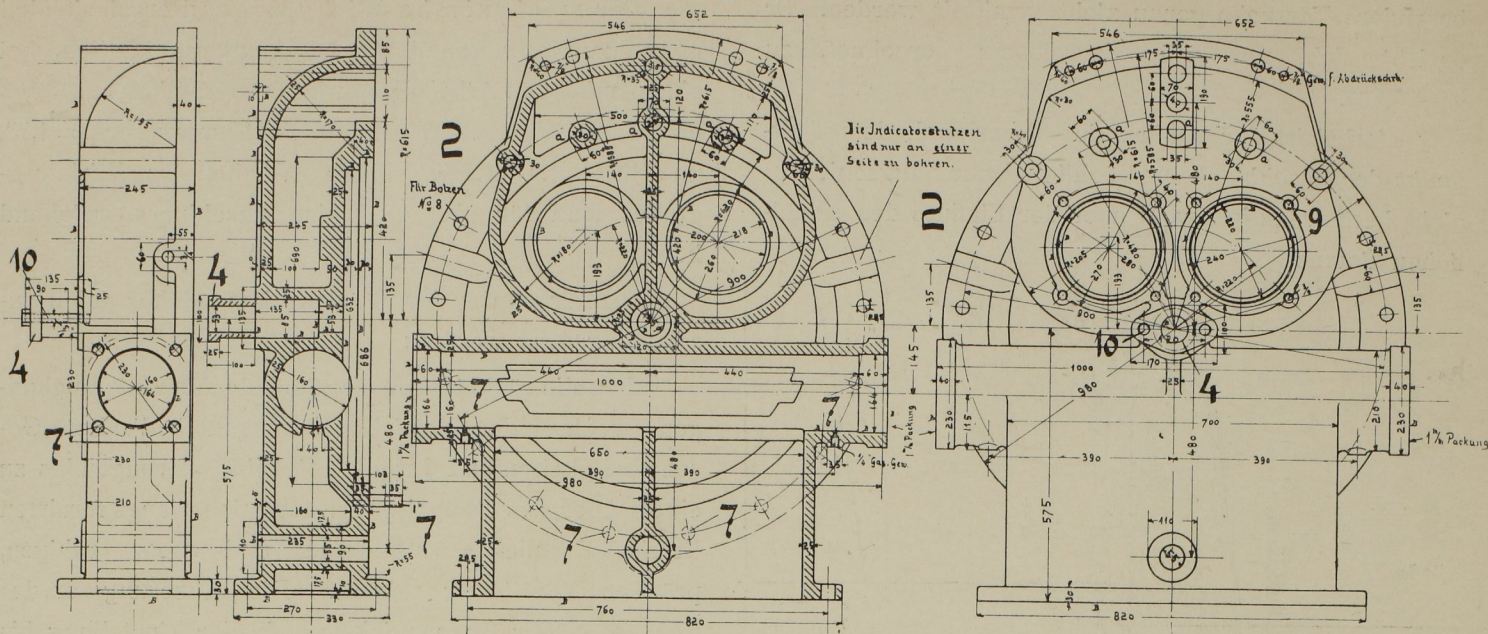
Abb. 23. Ventilkasten. Massst. 1:15.
