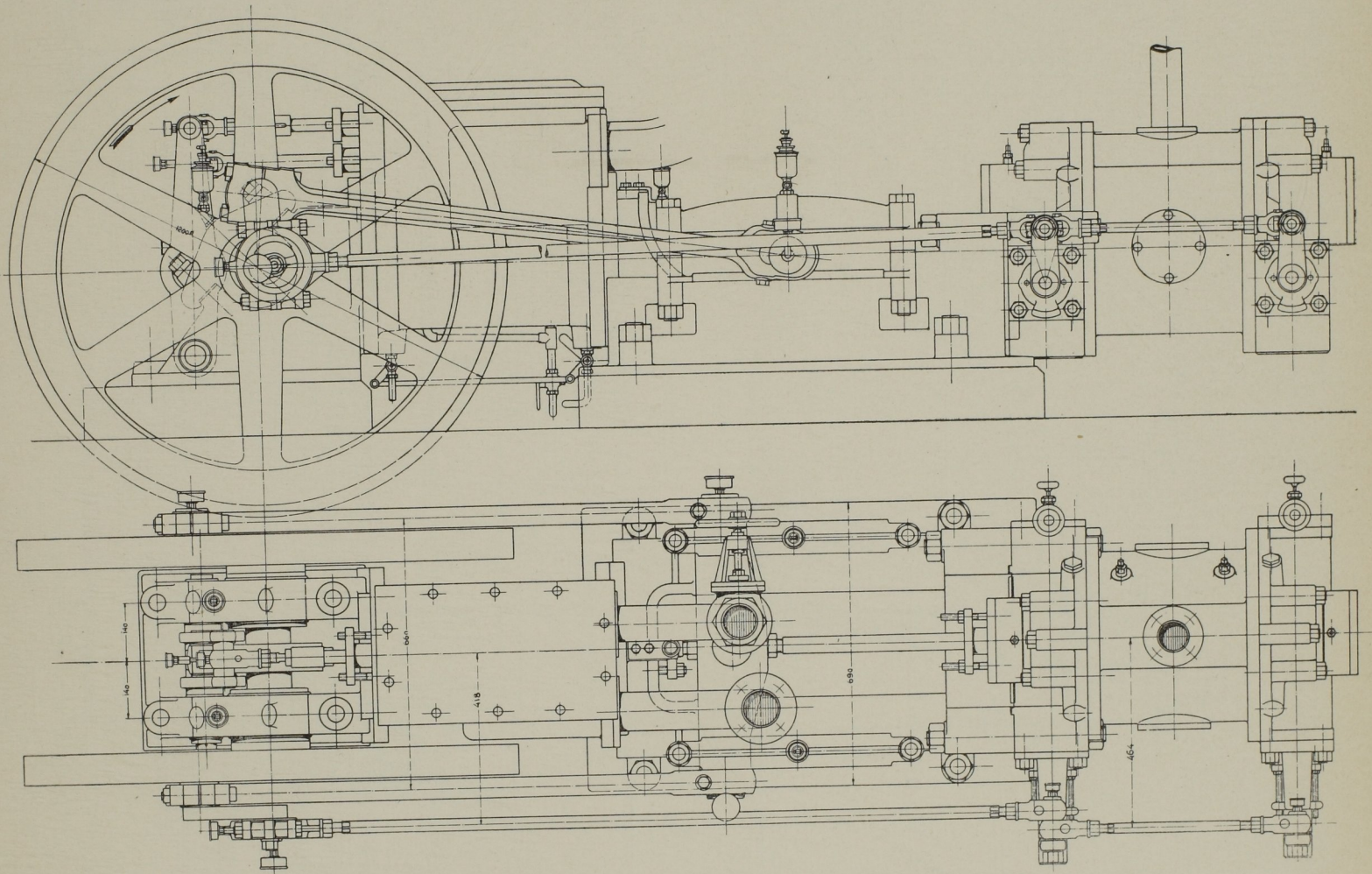
Abb. 1. Seitenansicht und Grundriss. Massst. 1:15.
