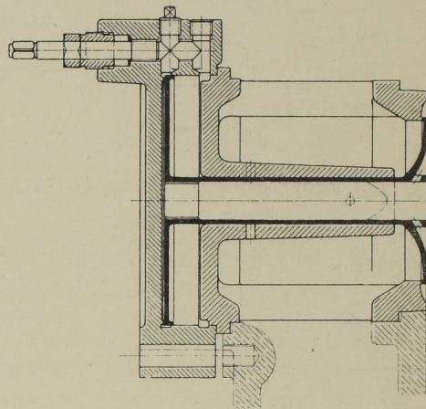
Abb. 25. Druckventil. Massst. 1:5.
