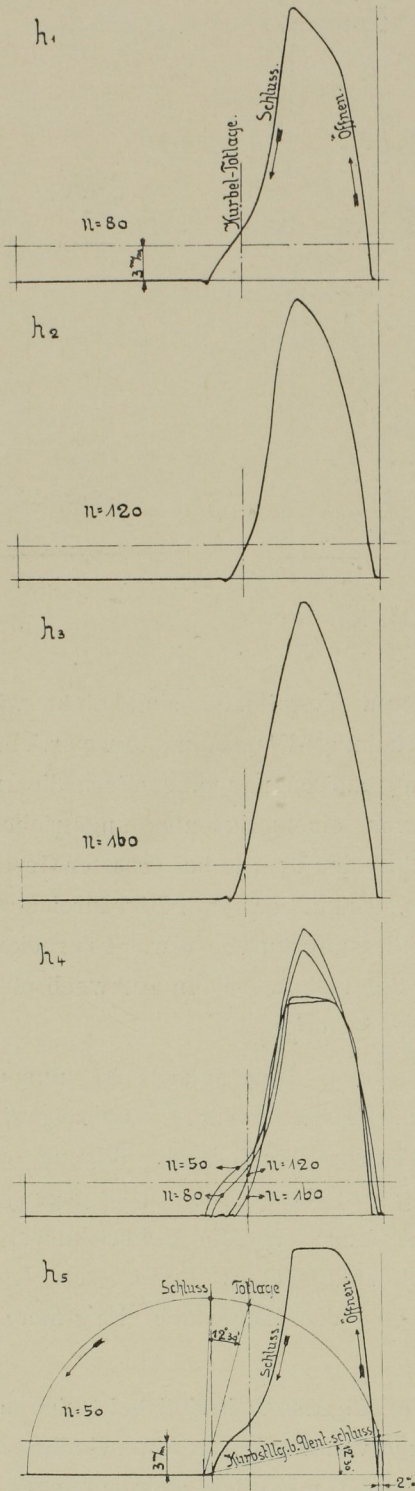
Abb. 18. Ventilhebungs-Diagramme.
