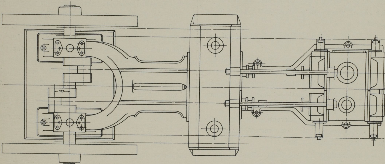
Abb. 9. Verbund-Kompressor mit rückläufigen Ventilen. Masst. 1:30.
