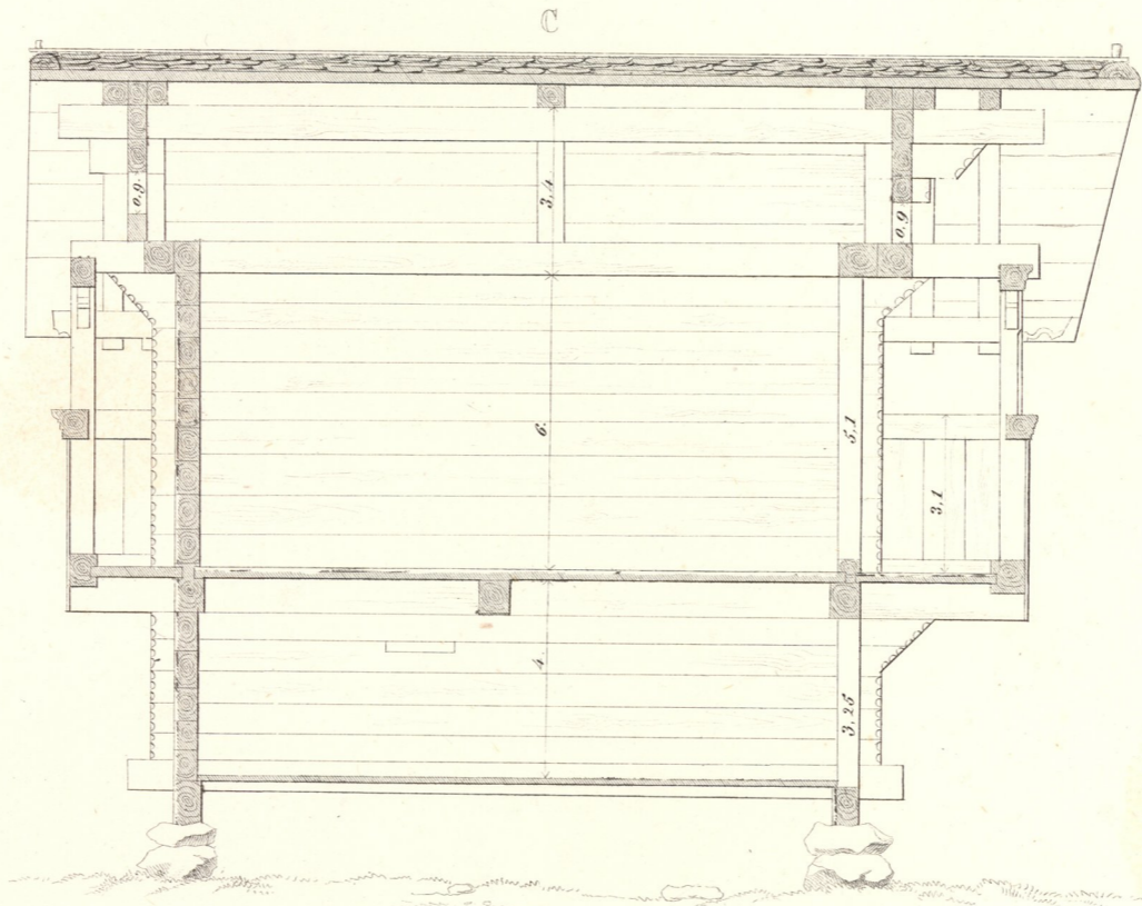
DURCHSCHNITT AUF DER LINIE A. B. DES PLANES. COUPE SUR LA LIGNE A. B. DU PLAN.
