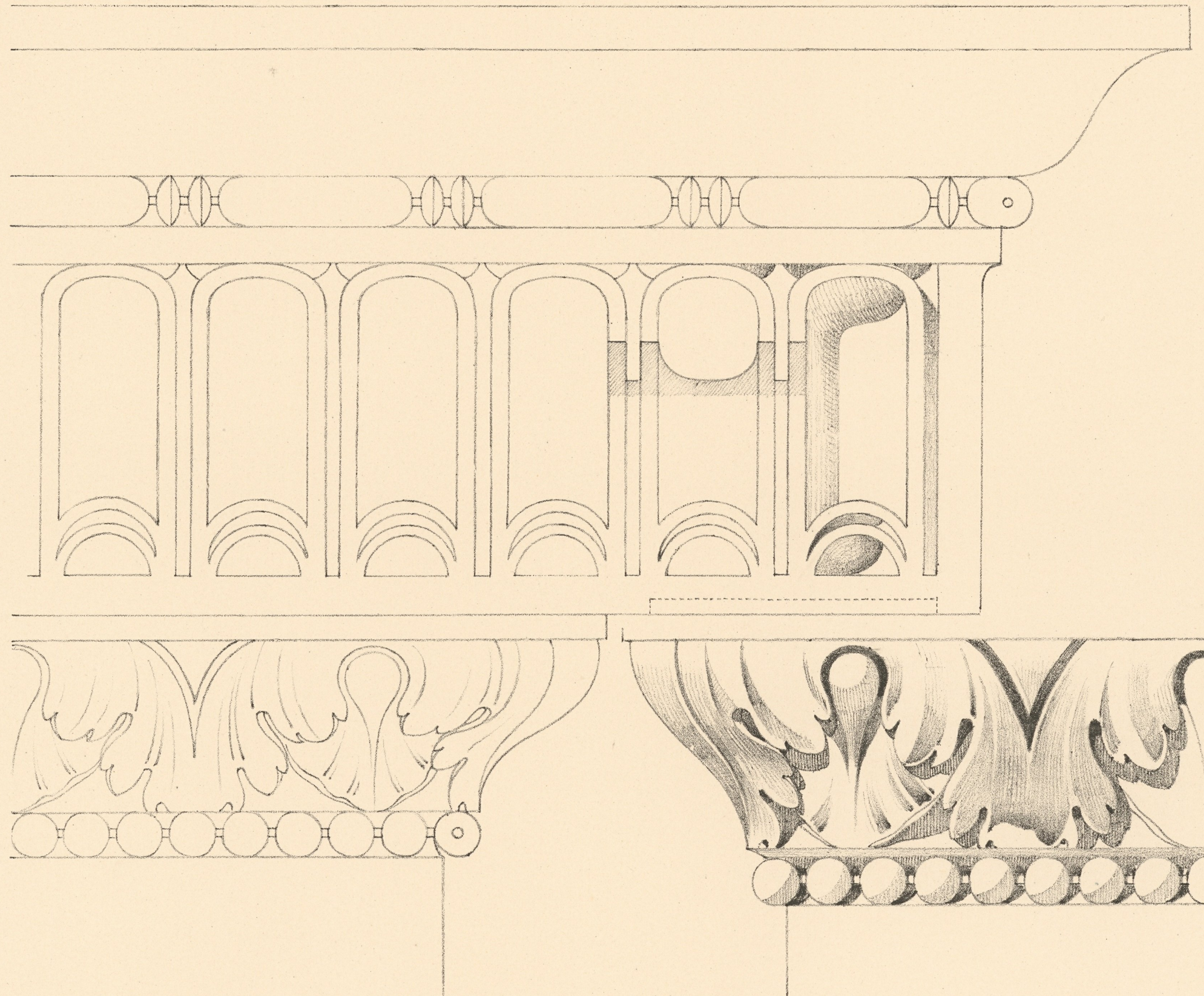
FENSTER-GESIMSE IM PARTERRE. (NATÜBL. GRÖSSE.)
