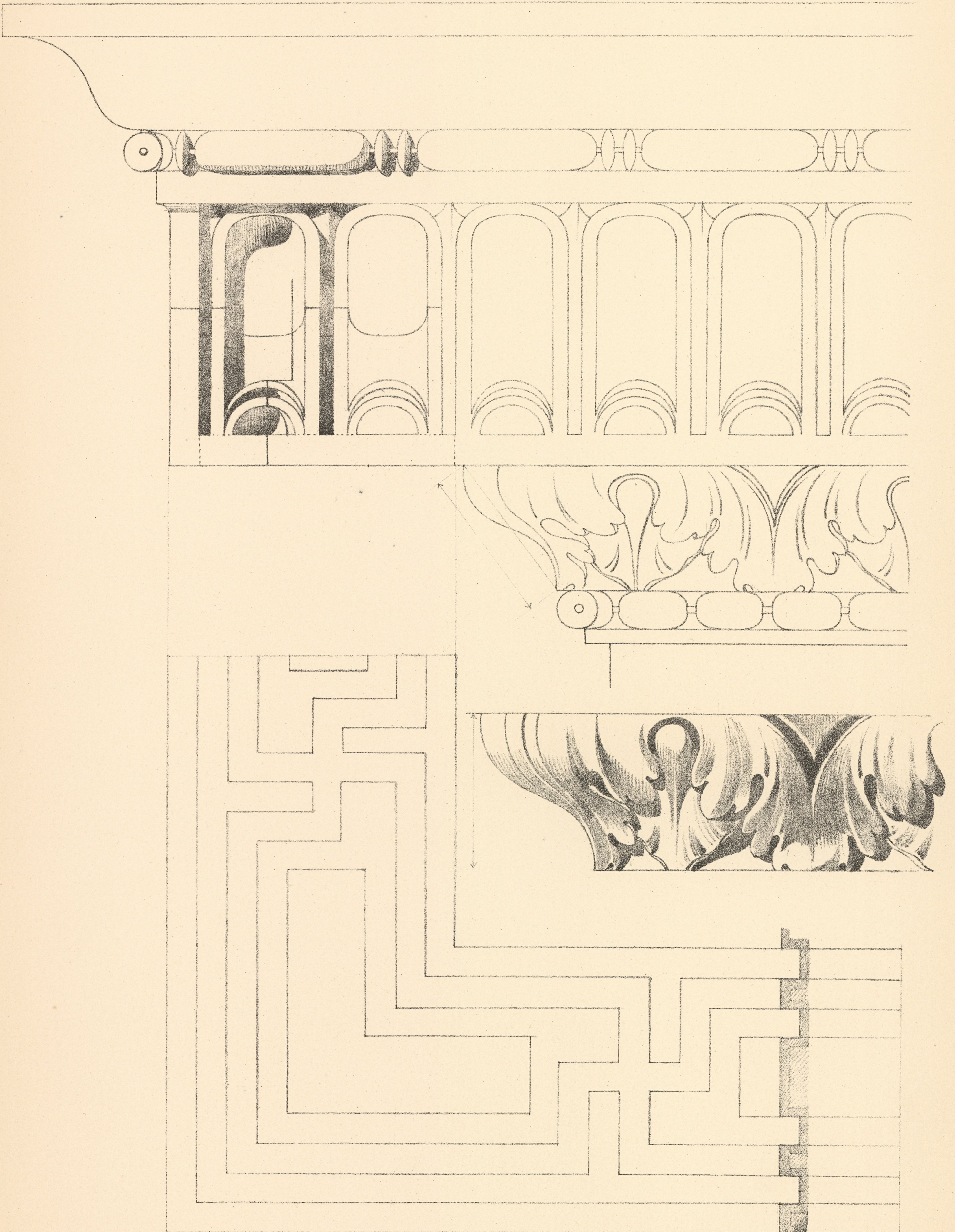
GESIMSE ÜBER DER THÜRENEINFASSUNG.
