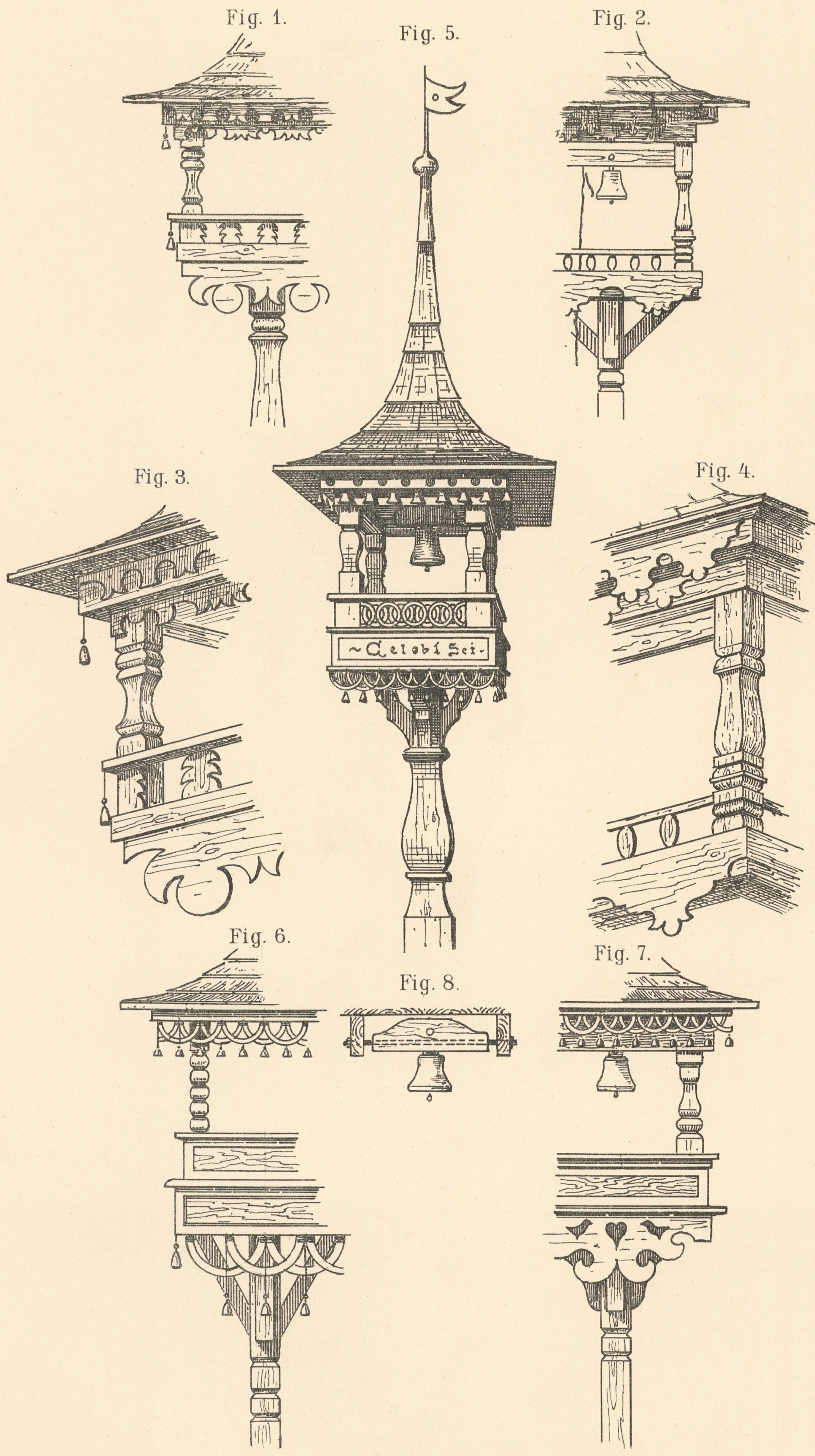
Masstab 1:20 für Fig. 1, 2, 5, 6 u. 7.
