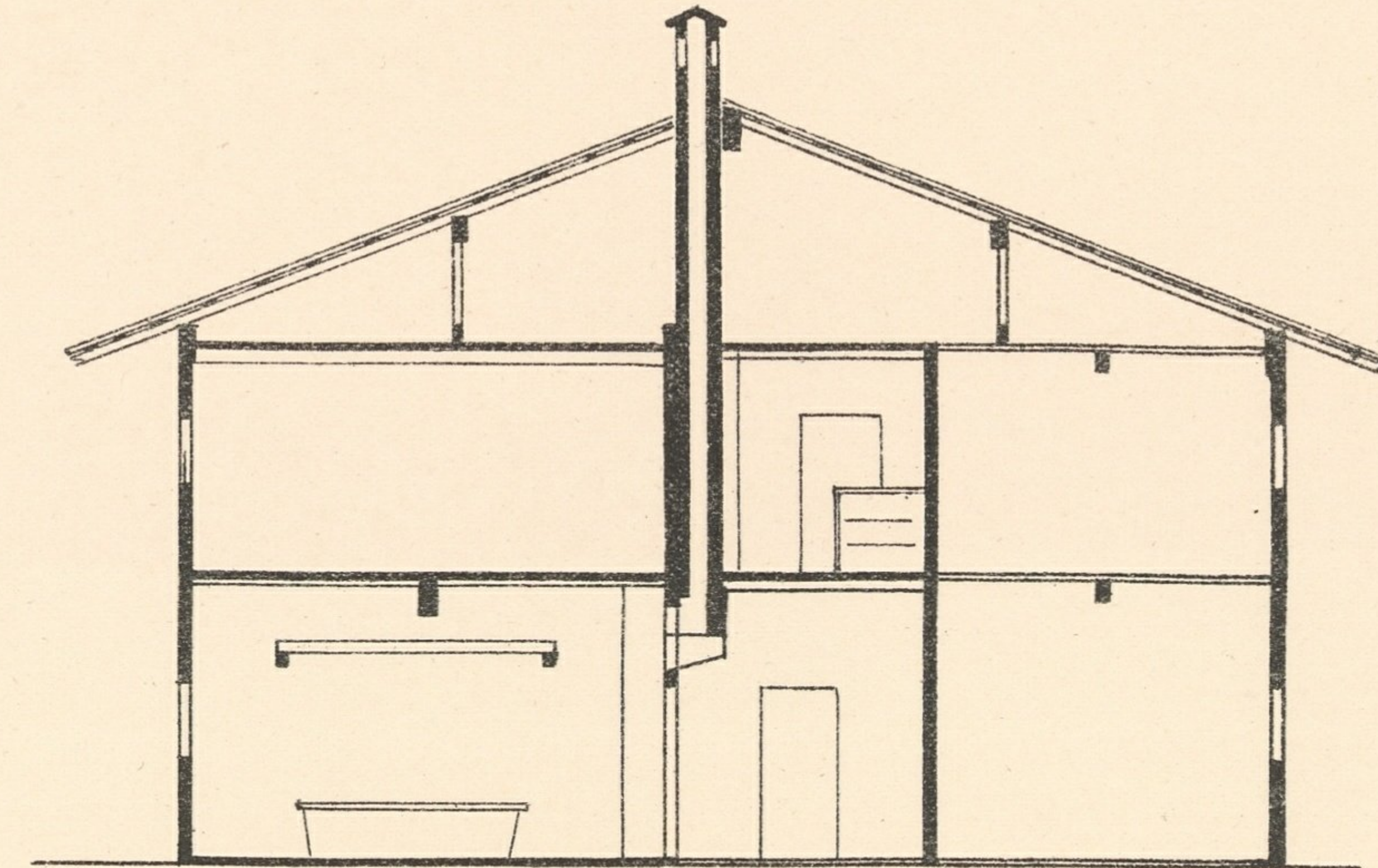
Schnitt SS.
