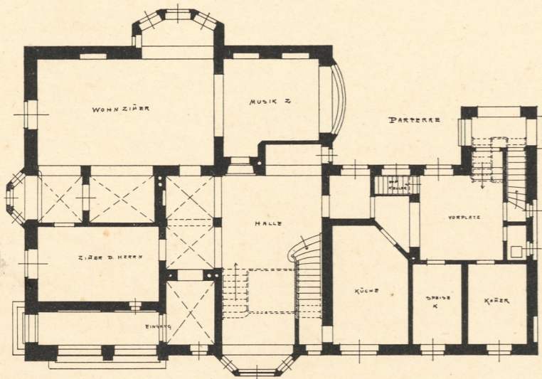
Zu Tafel 27: Wohnhaus Arthur Riemerschmid in Pasing.
