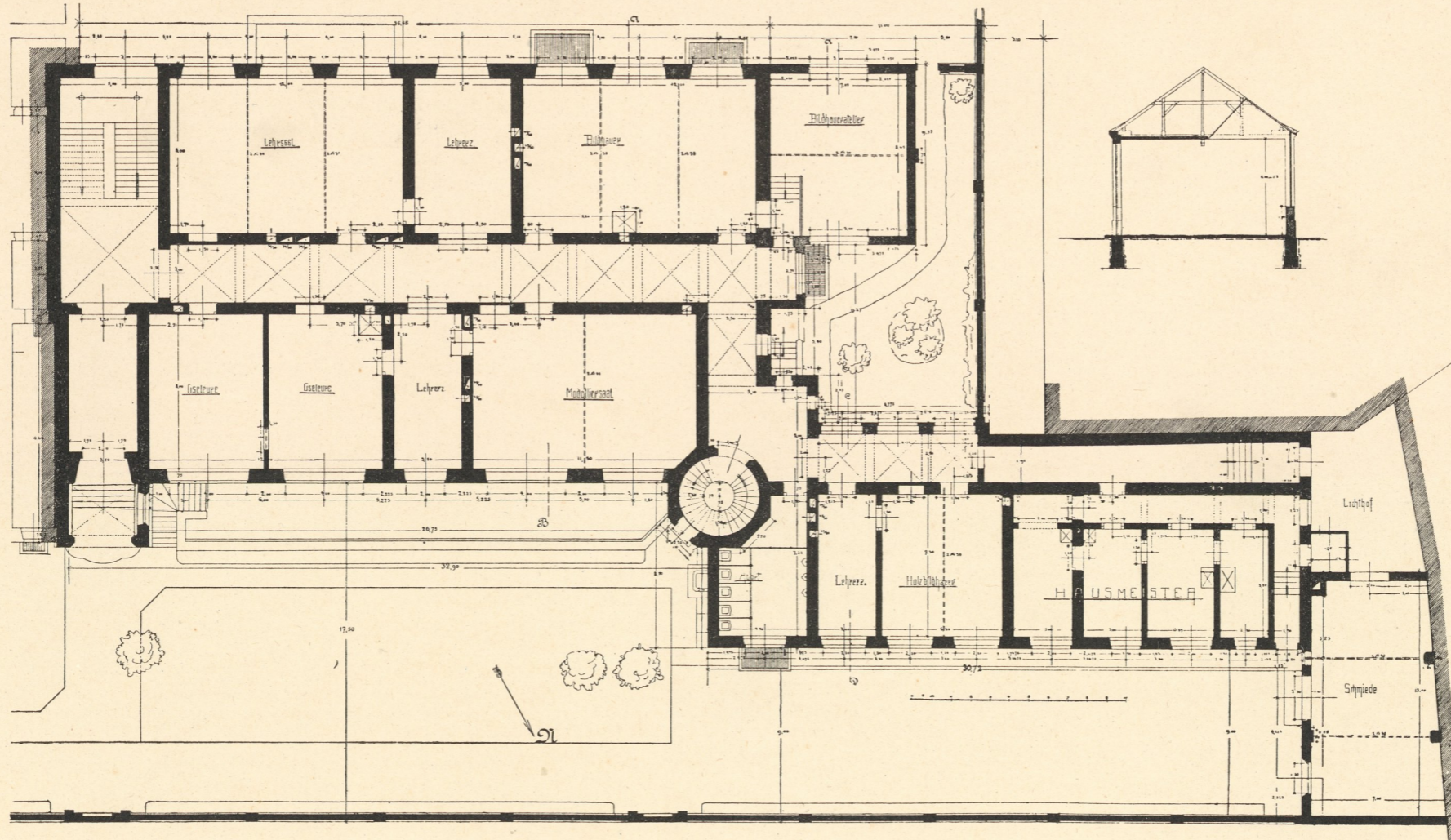
Zu Tafel 18: Städtische Gewerbeschule an der Louisenstrasse.
