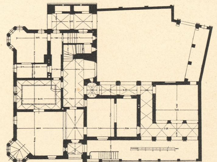
Zu Tafel 28: Wohnhaus E. Riemerschmid in Starnberg.
