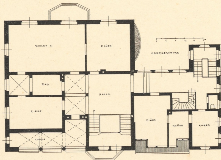
Zu Tafel 27: Wohnhaus Arthur Riemerschmid in Pasing.
