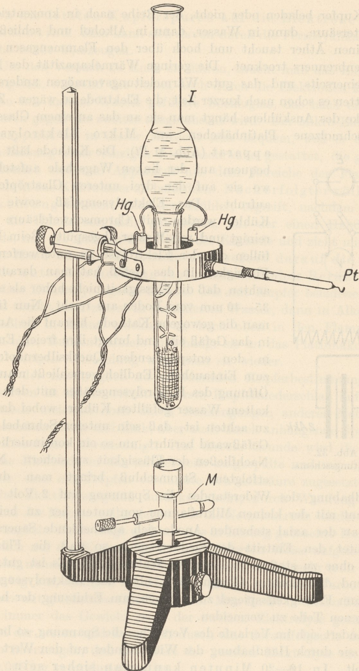
Abb. 31. Apparat z. Ausführung d. elektroanalyt. Kupferbestimmung. ( \frac{1}{2} nat. Größe.) I Innenkühler, Hg Quecksilbernäpfchen, Pt Platinhäkchen, M Mikrobrenner.
