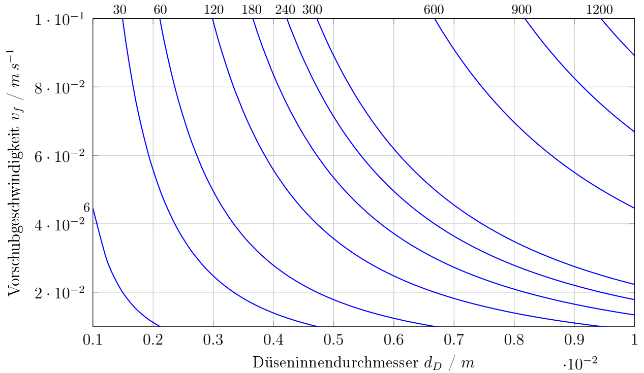
Abbildung 4.55: Bestimmung des Volumenstrom Q_P in ml \cdot min^{-1} bei tropfenartiger Oberflächenstruktur (Quelle: Eigene Darstellung)
