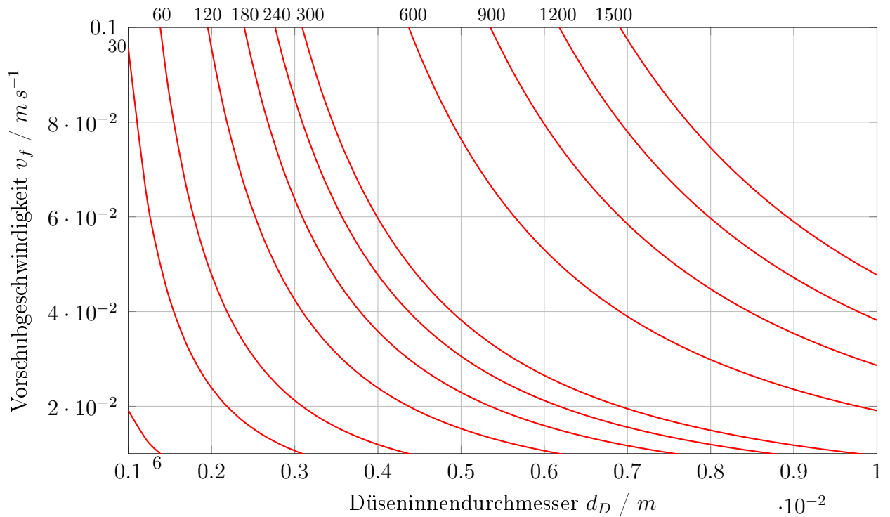
Abbildung 4.56: Bestimmung des Volumenstroms Q_P in ml \cdot min^{-1} bei strahlartiger Oberflächenstruktur (Quelle: Eigene Darstellung)
