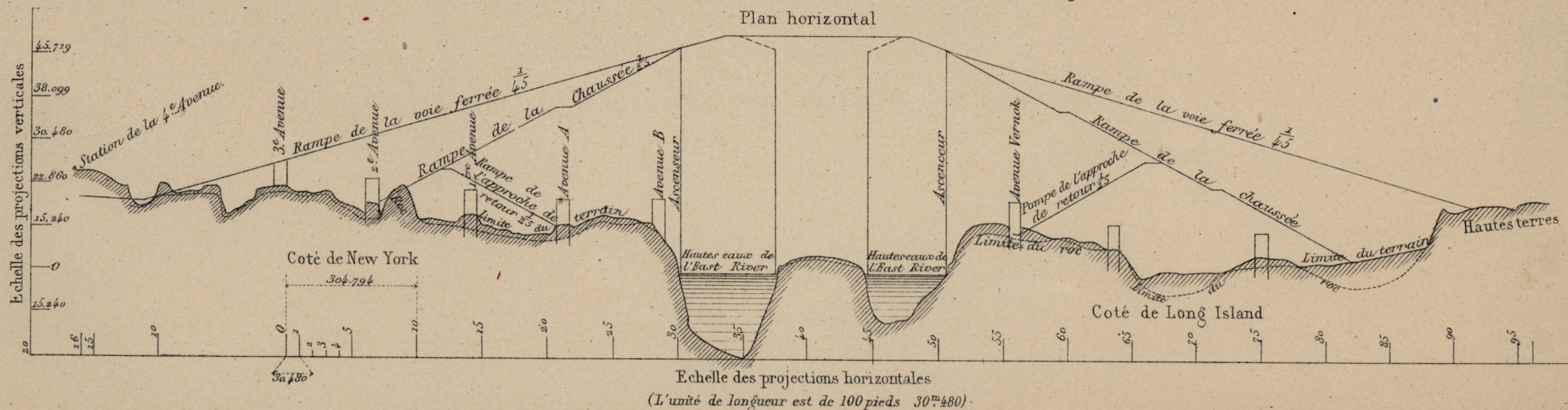
Fig. 5. Profil des rampes du pont projeté entre New York et Long Island
