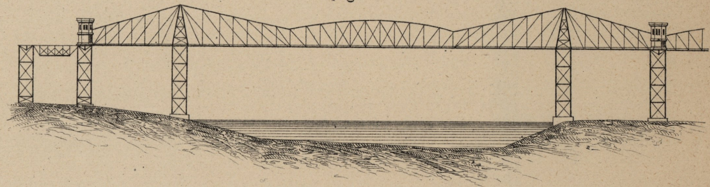
Fig. 4. Ensemble du projet de M. C. O. Brown (Compagnie de Passaic)
