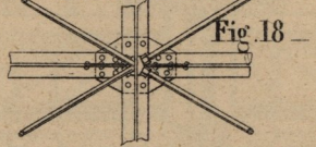
Plan des contreventements horizontaux.
