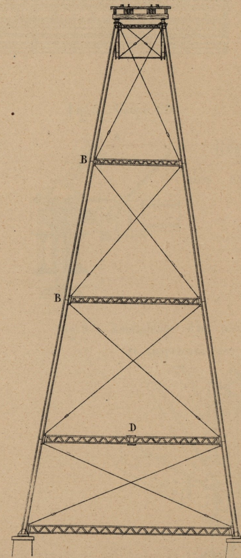
Fig. 3. — Coupe transversale.
