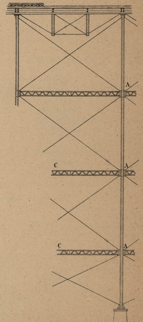
Fig. 4. — Elevation longitudinale.
