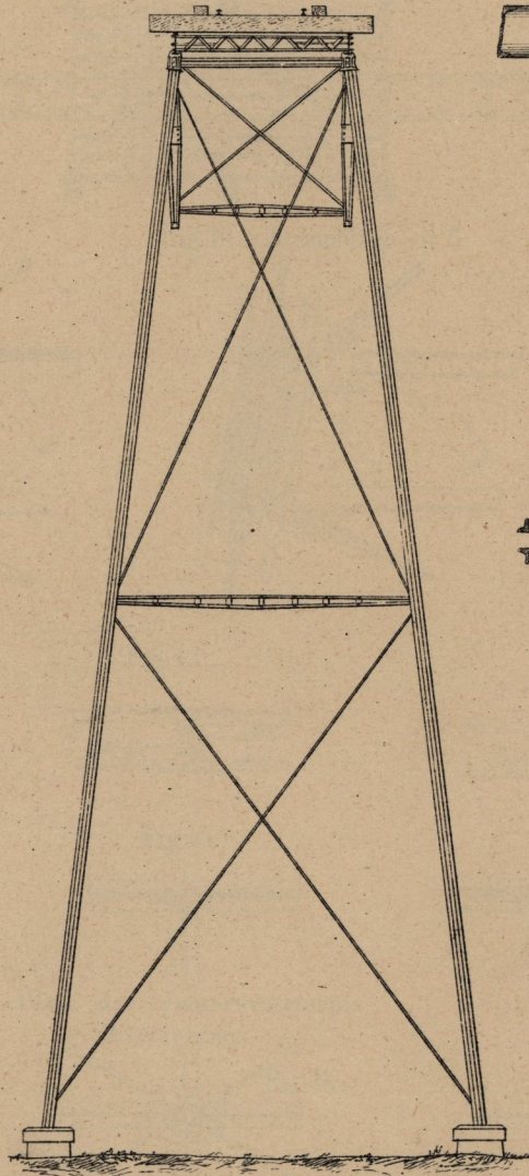
Fig. 3. Vue par bout.
