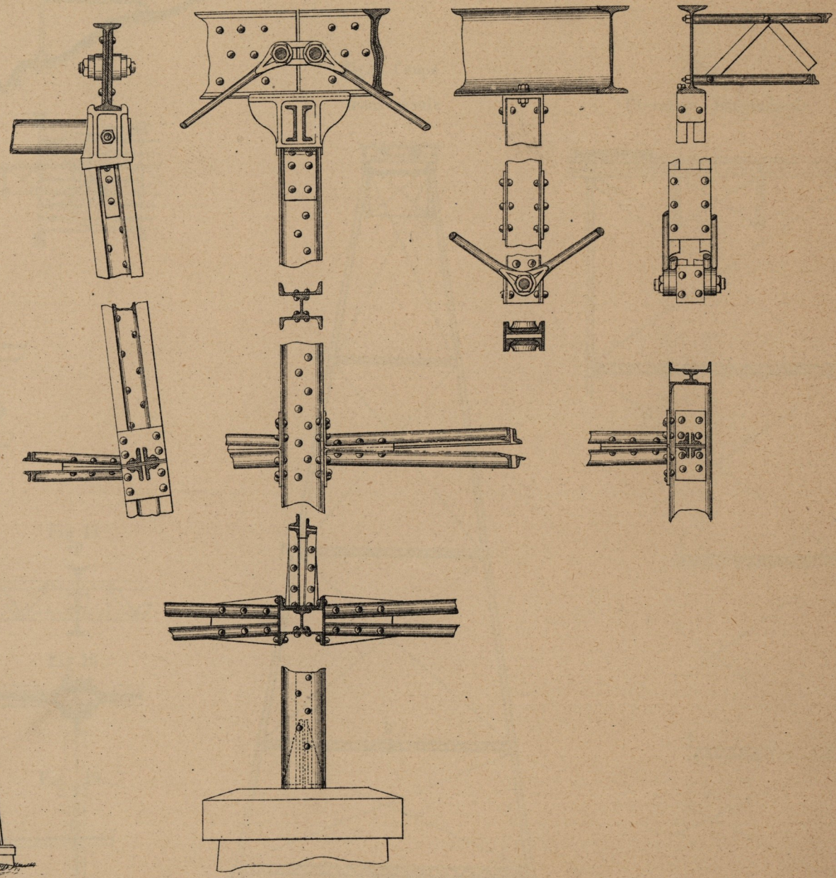
Fig. 4. Détails d'une pile. Echelle de 16
