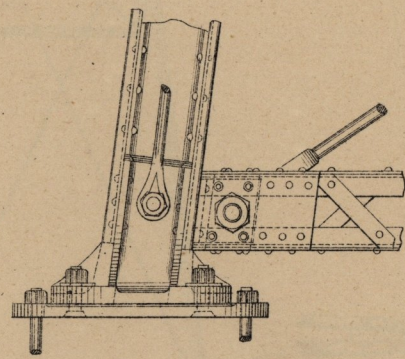
Fig.5 - Base des Piles
