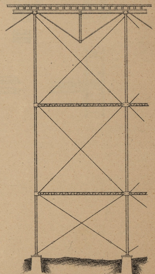
Fig.4 - Vue latérale.
