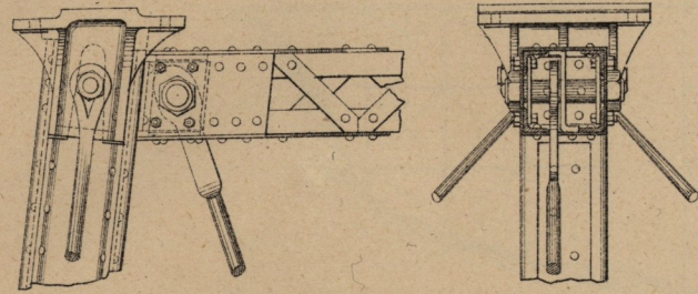
Fig.6 - Sommet des Piles.
