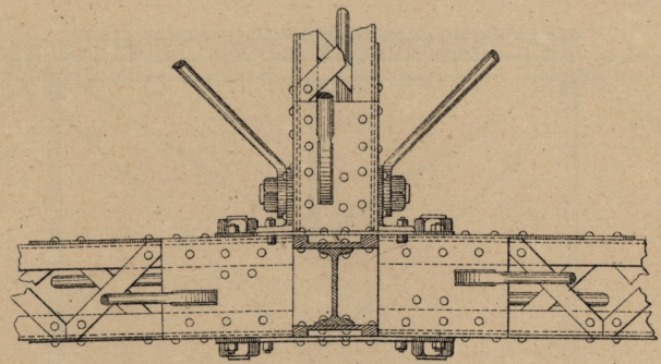
Fig.7 - Assemblages des piles avec les poutres transversales.
