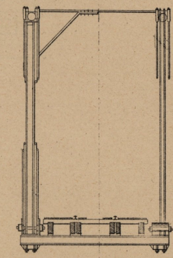
Fig. 5 - Coupe en travers.
