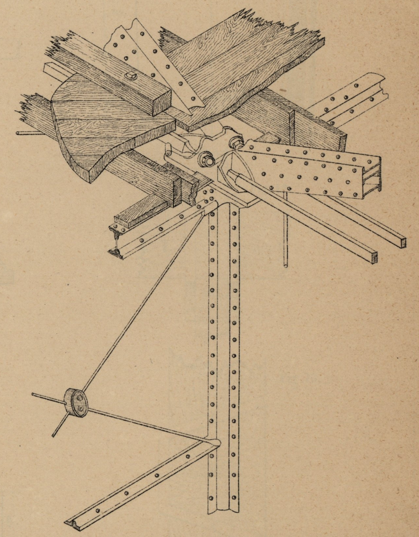
Fig. 3 — Détails des sabots des arcs en I.
