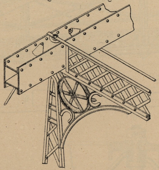
Fig. 7 — Assemblage de la corde inférieure et d'un montant
