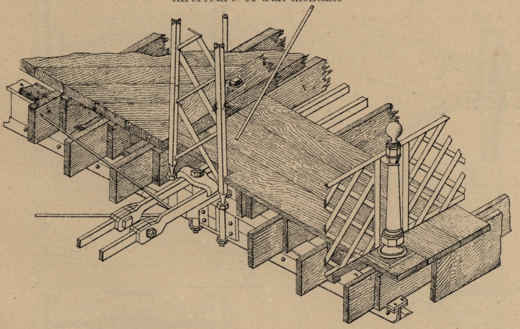
Fig. 7 — Assemblage de la corde inférieure et d'un montant
