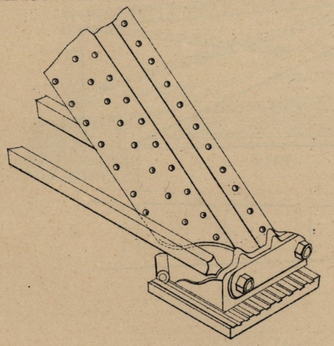
Fig. 2 — Sabot extrême
