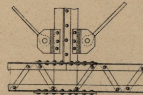
Poutre longitudinale intermédiaire
