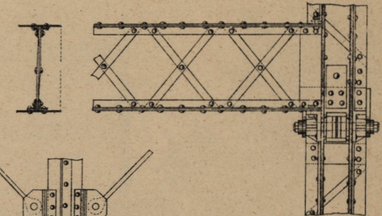
Pièce longitudinale
