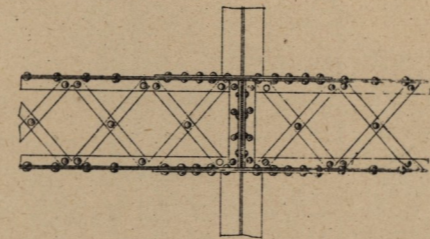
Pièces verticales au milieu des piles dans le sens transversal Assemblages avec les pièces horizontales
