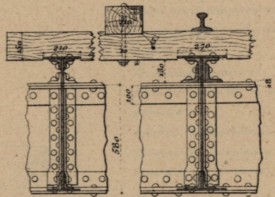
Fig.18 - Coupe OP
