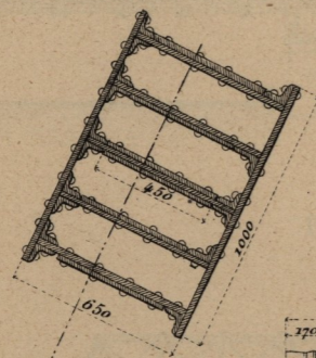
Fig.15 - Coupe GH
