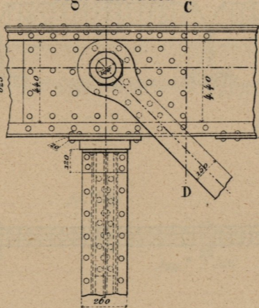
Fig.3 - Elevation c
