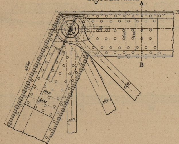
Fig.1 - Elevation
