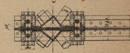
Fig. 21. Coupe RS
