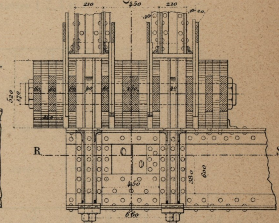
Fig. 21. Coupe RS
