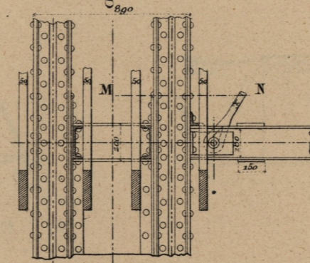
Fig.9 - Coupe MN
