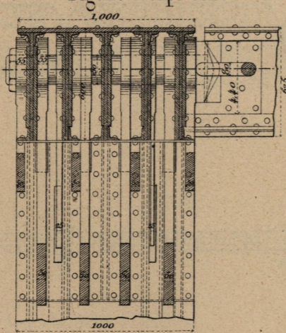
Fig.2. Coupe AB.
