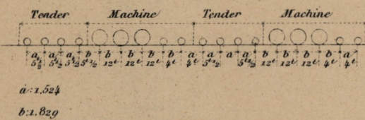
Fig. 4 - Distribution du poids roulant
