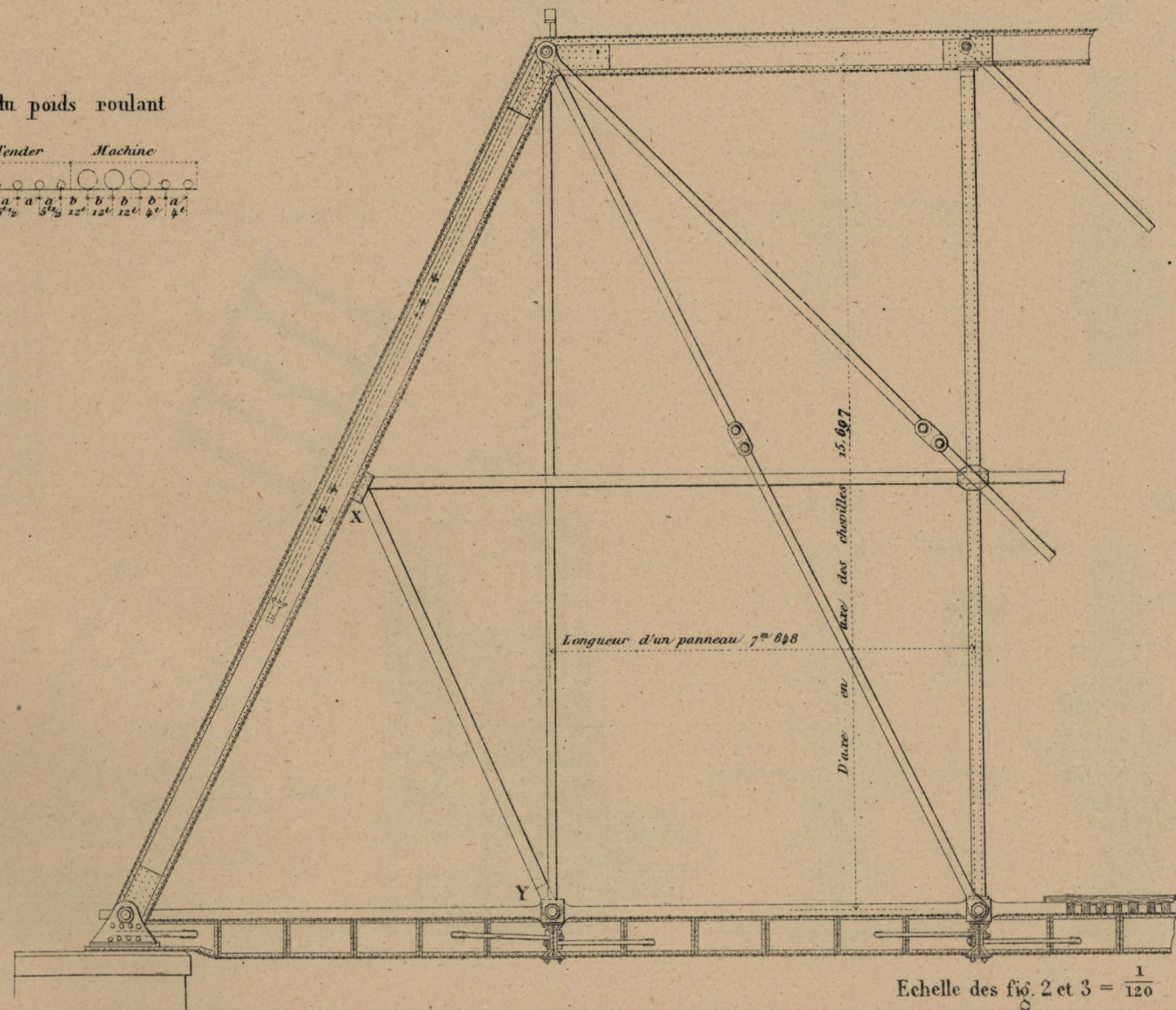
Fig. 2 - Détail à l'extrémité de la travée
