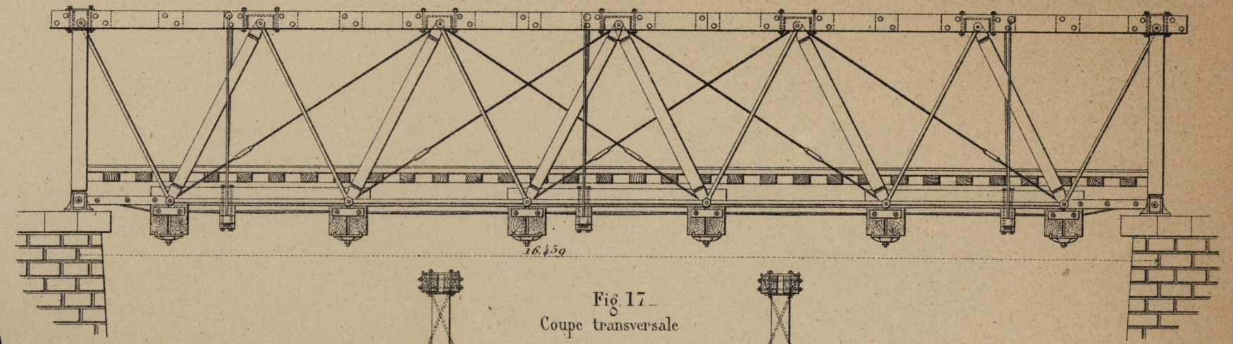
Pont sur le Missouri. (Chemin de fer du Pacifique) Fig. 16 - Elevation. Fig. 17 - Coupe transversale
