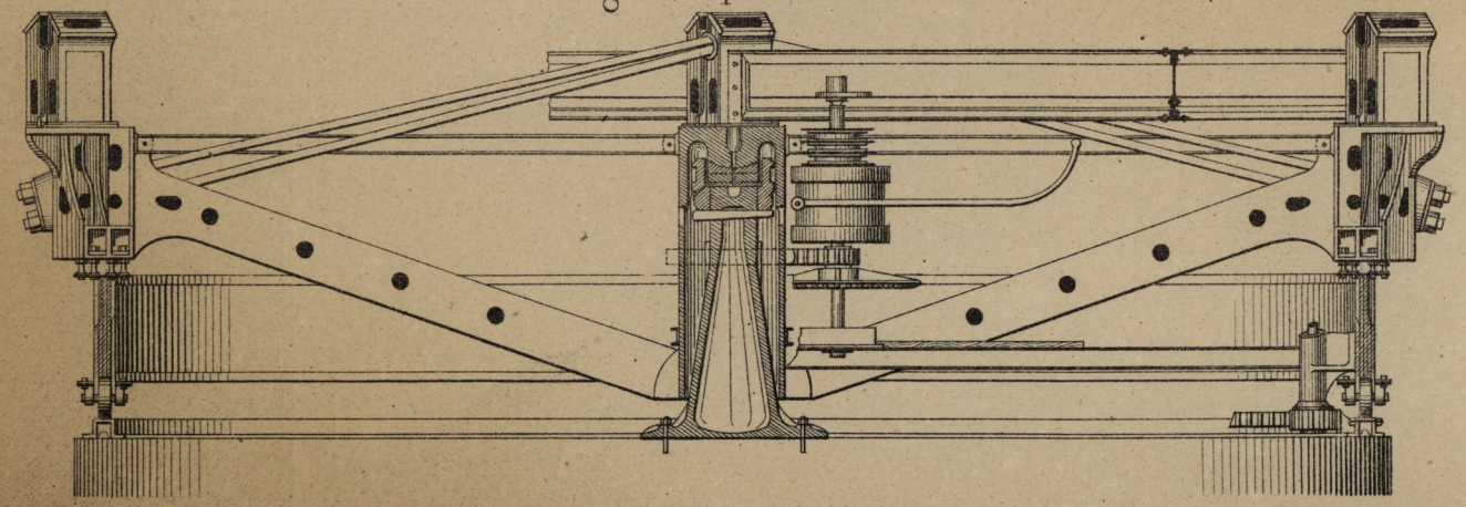
Fig. 15 - Coupe diamétrale.
