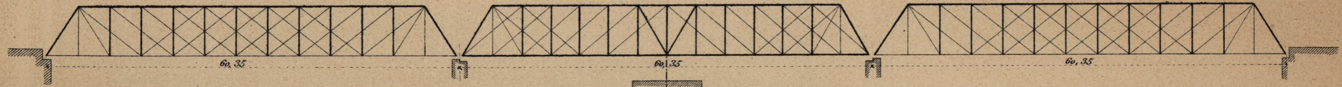
Fig.2 Elevation de la travée tournante.
