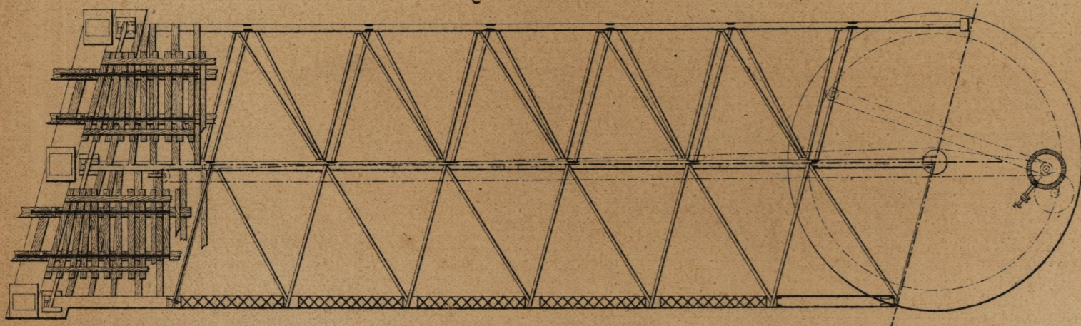
Fig.5 Demi-élévation d'une travée fixe.
