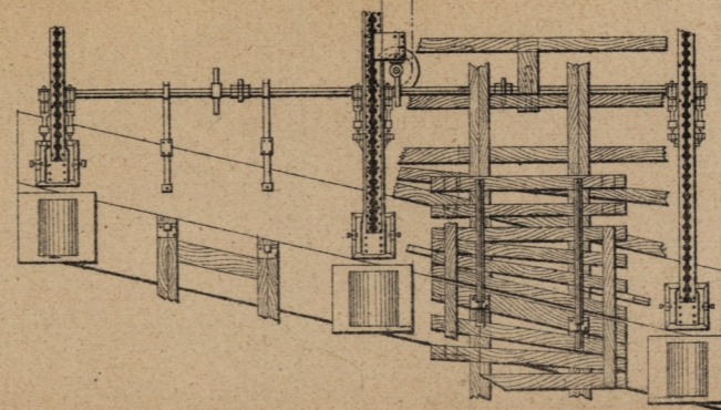
Fig.6 Plan à l'une des piles extrêmes de la travée tournante.
