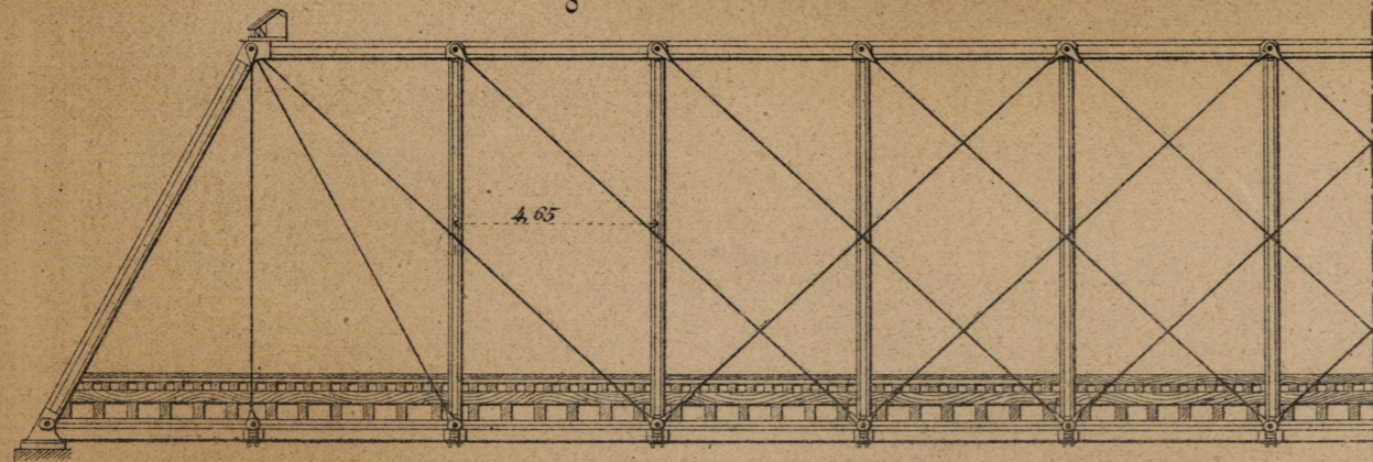
Fig.5 Demi-élévation d'une travée fixe.
