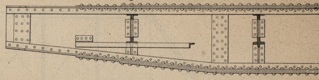
Fig. 4_Poutre du plancher
