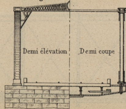
Fig. 3_Vue transversale
