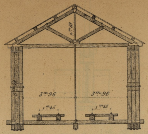
Fig. 1. Coupe transversale
