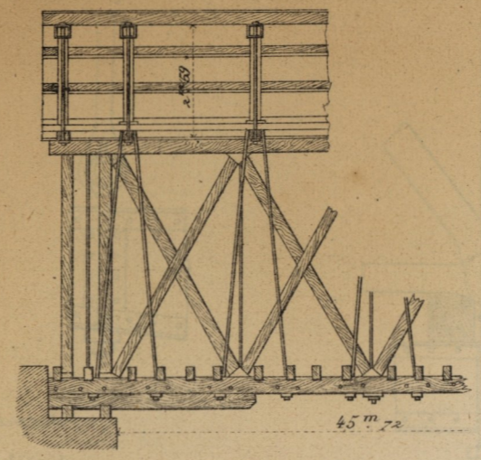
Fig. 2. Coupe Longitudinale
