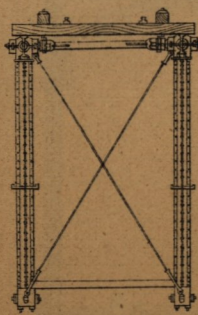
Fig.3 Coupe CD
