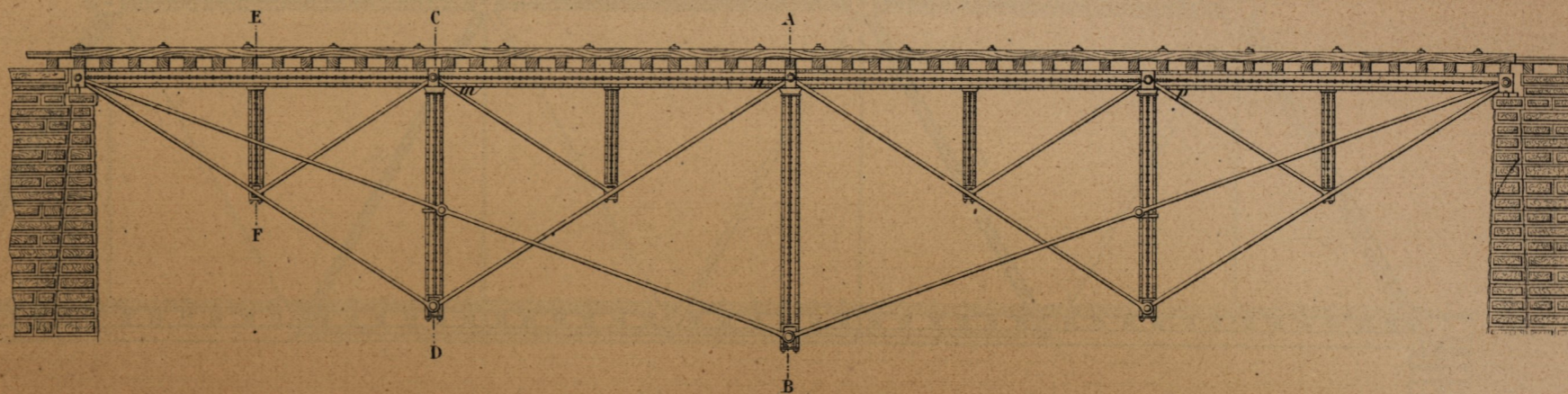
Fig.2 Plan d'ensemble
