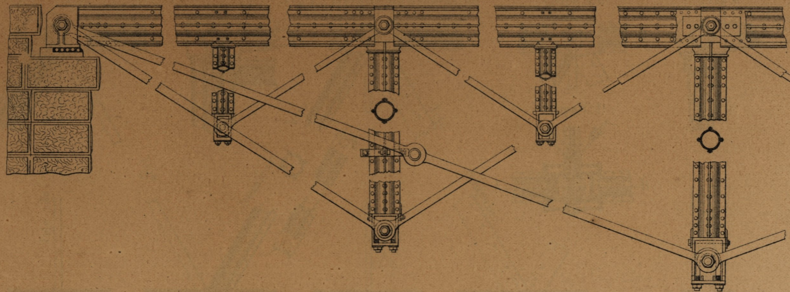
Détails de l'Elevation
