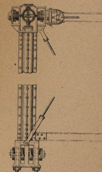
Demi-coupe transversale au milieu
