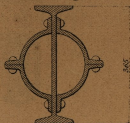
Fig.8 Section de la corde supérieure
