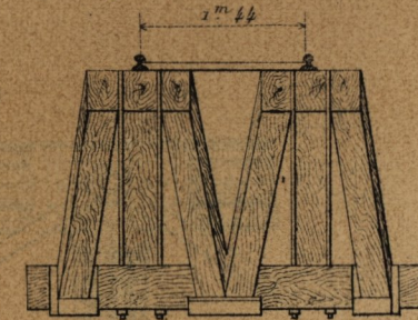
Fig 6. Coupe transversale
