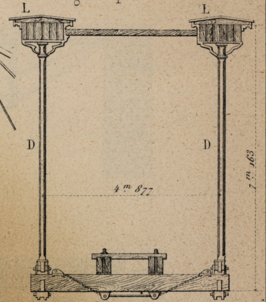
Fig 2. Coupe en travers
