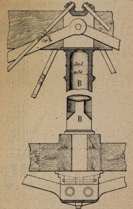
Fig 4. Montant du milieu Elevation laterale
