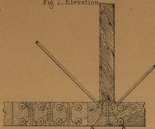
Fig. 6 et 7. Détail de l'assemblage A
