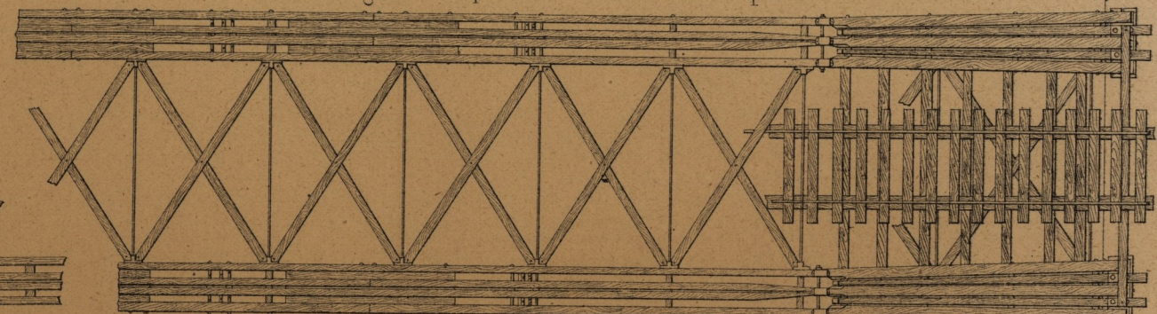
Détail en B. Fig. 8
