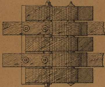
Fig. 4 et 5. Assemblage du dernier bras. avec la corde inférieure
