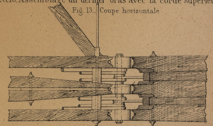
Fig. 12 et 13. Assemblage du dernier bras avec la corde supérieure
