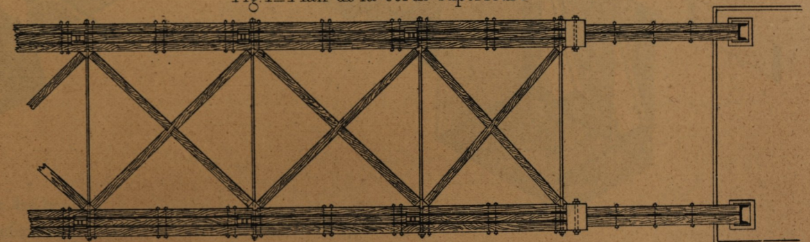
Fig 4 - Plan de la corde supérieure
