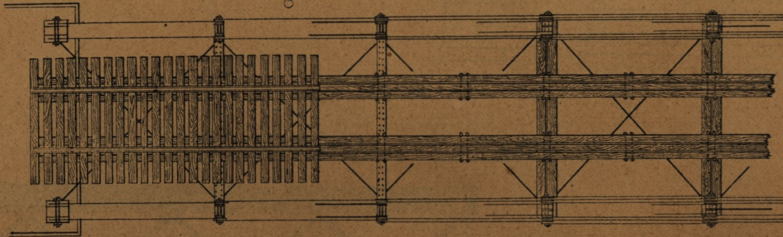
Fig 3 - Plan de la corde inférieure
