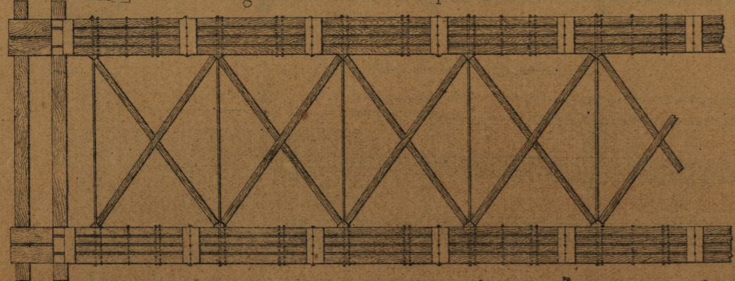
Fig. 3 Plan de la corde supérieure
