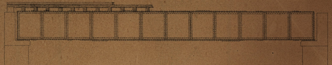
Fig. 11. Elevation
