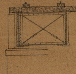
Fig. 13. Coupe transversale
