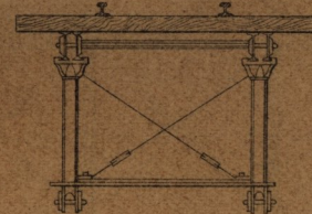
Fig. 10. Coupe transversale
