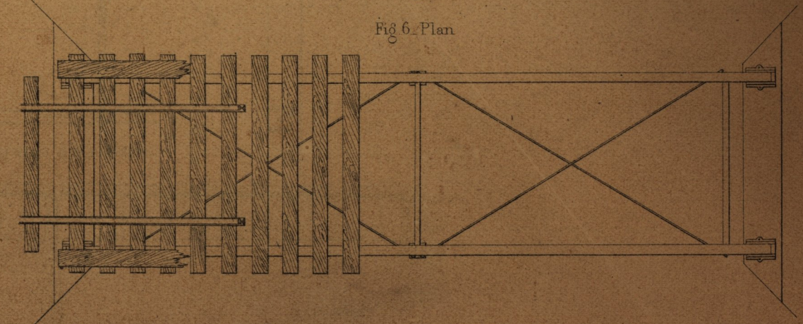
Poutre pleine pour les portées de 8 à 20 mètres.
