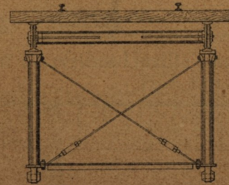
Fig. 7. Coupe transversale
