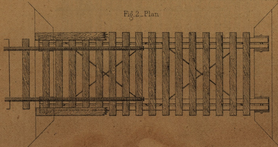
Poutre armée pour portées de 8 à 13 mètres.
