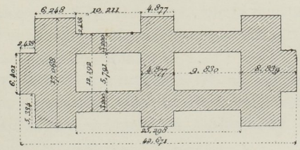
Fig. (10). Plan d'une tour.
