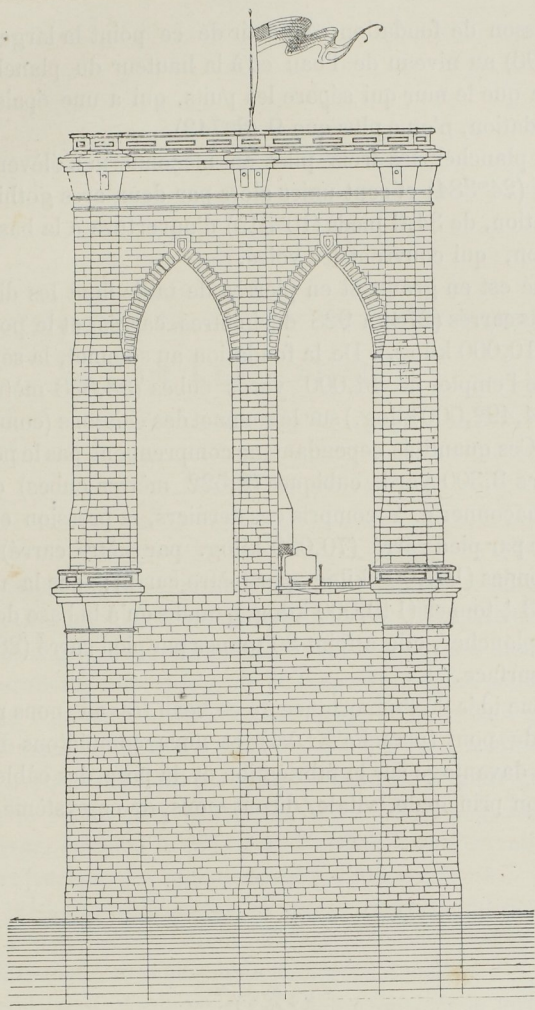
Fig. (9). Elévation d'une tour.
