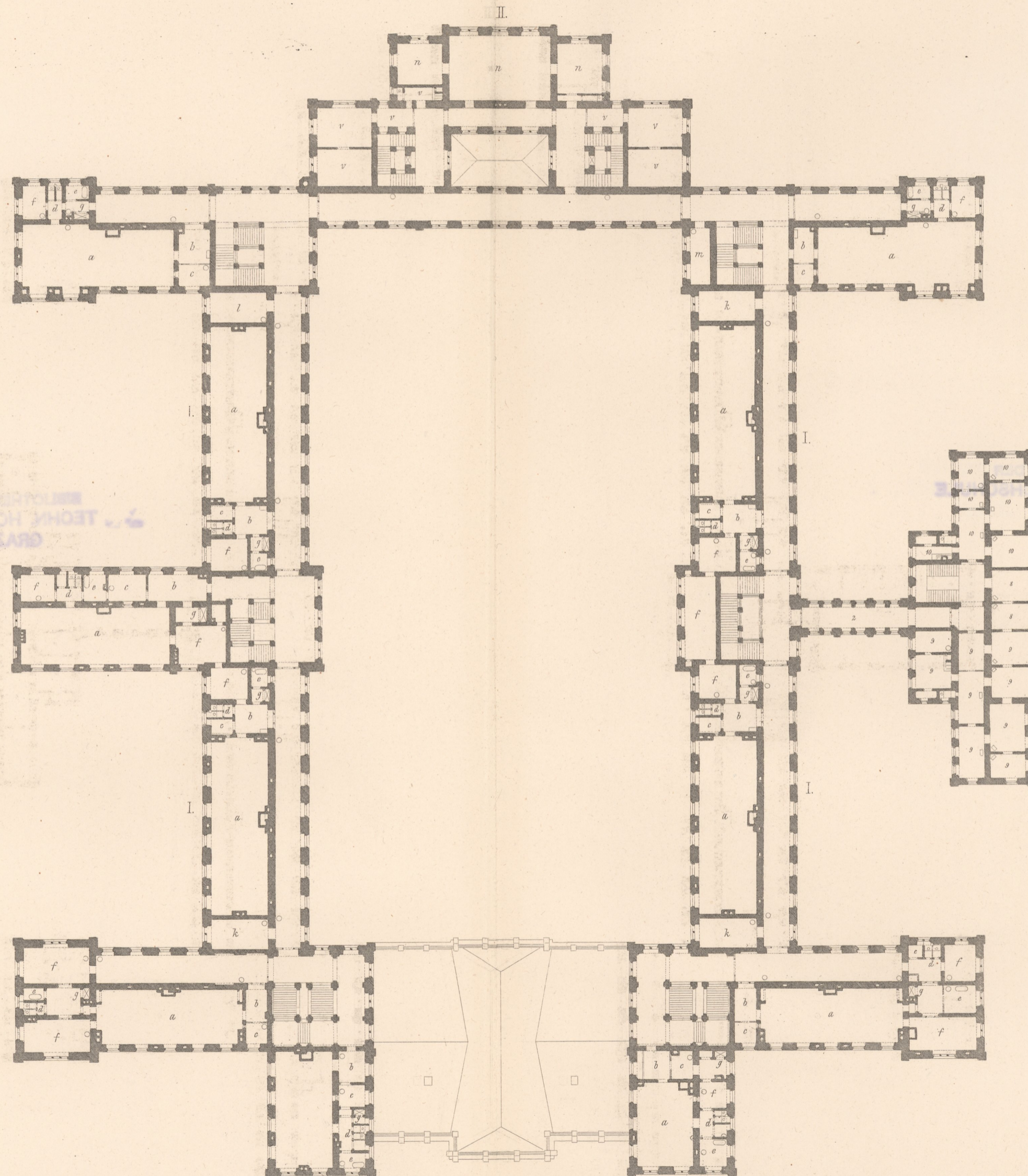
Grundriss des 1 ten Stockes.
