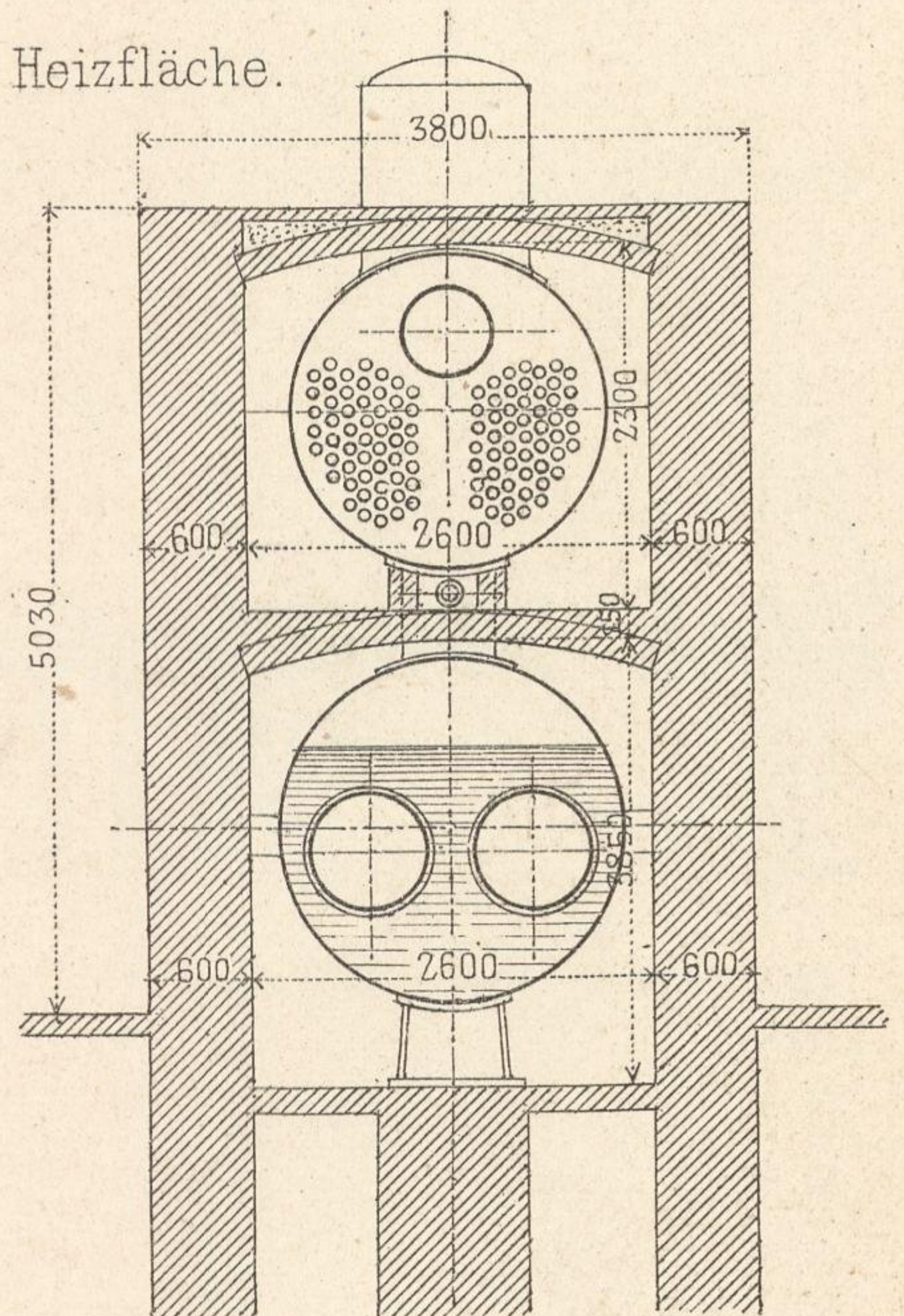
Fairbairnkessel, 160 m 2 Heizfläche.
