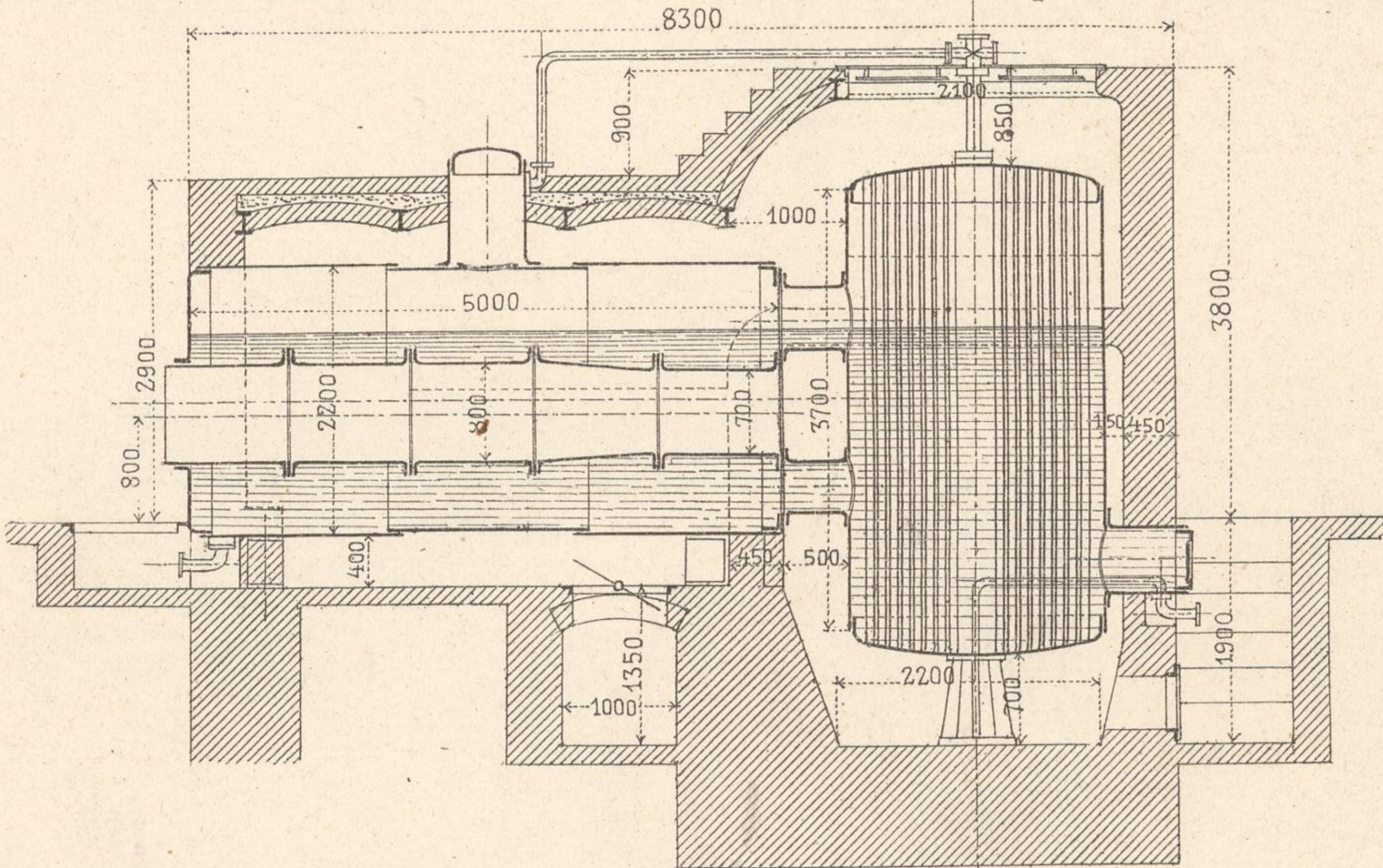
Tischbeinkessel, 200 m 2 Heizfläche.
