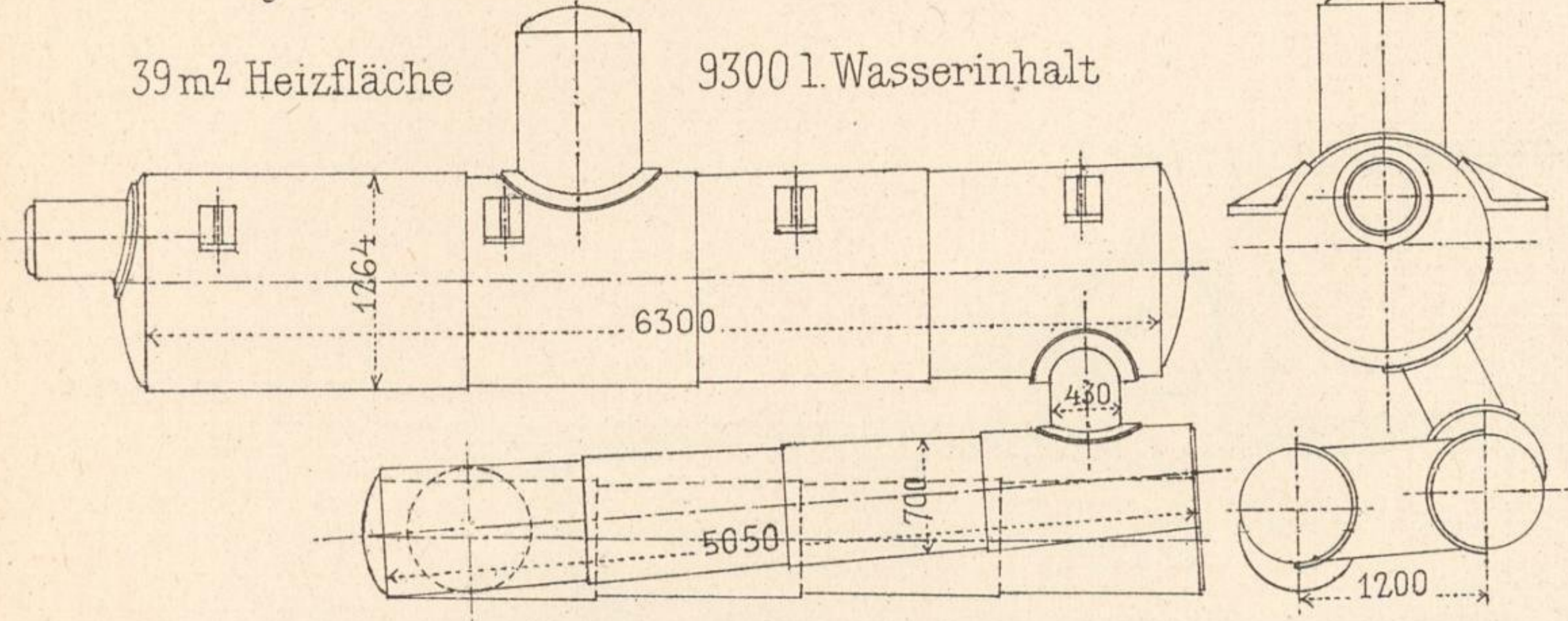
Cylinderkessel mit 2 Unterkesseln
