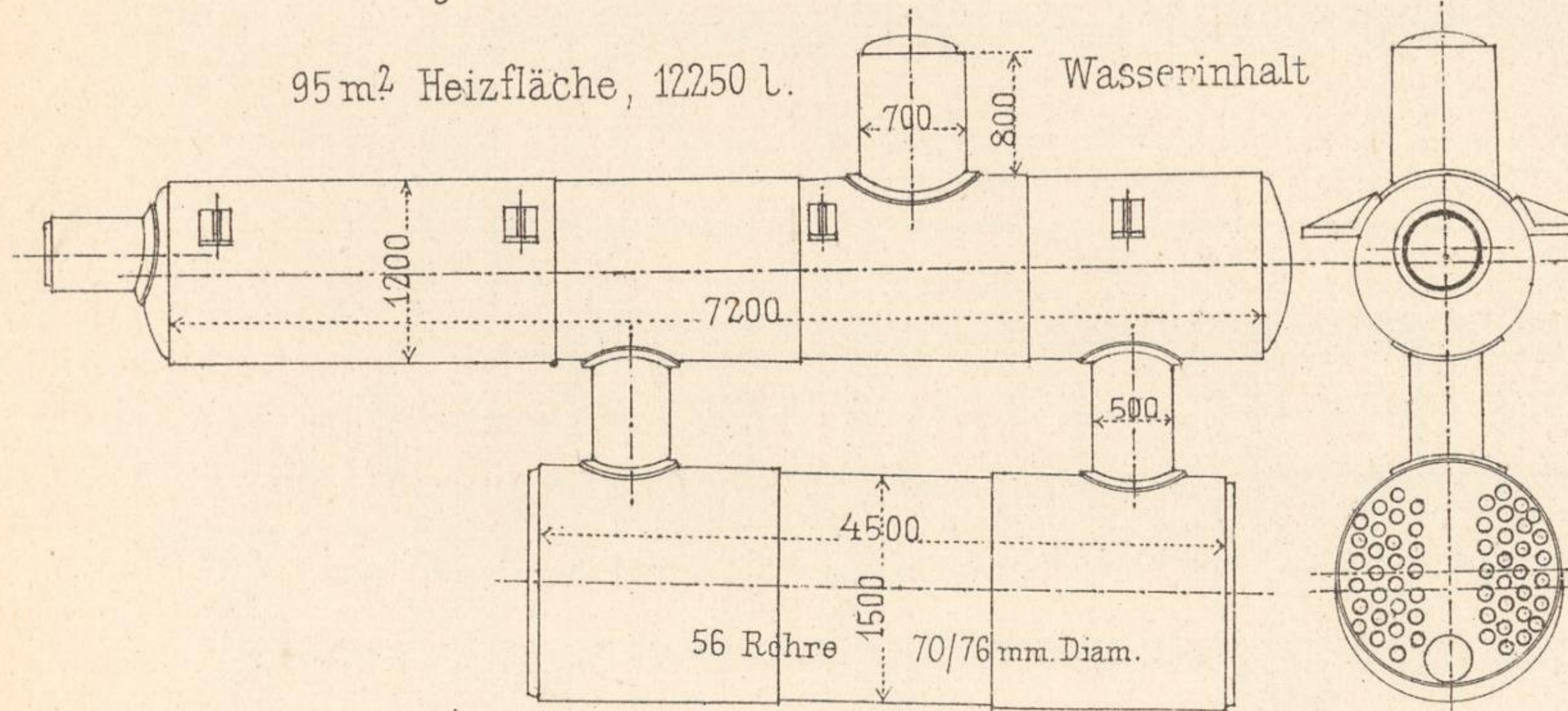
Cylinderkessel mit Röhrenkessel.
