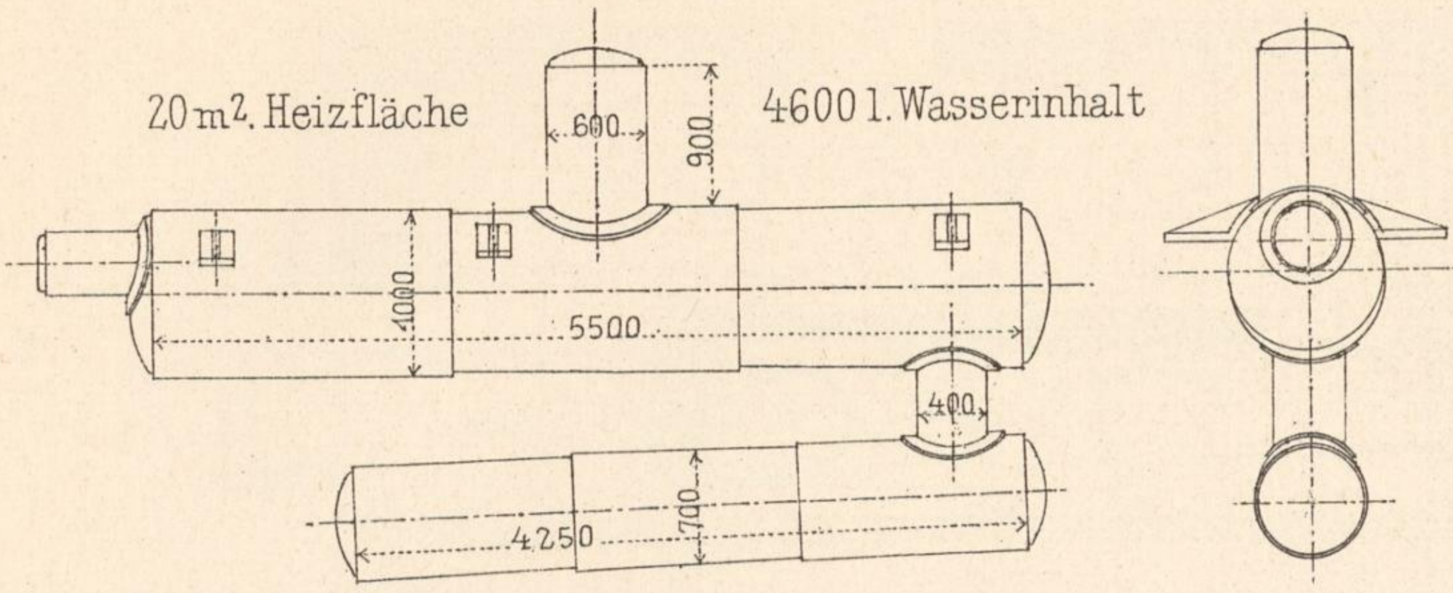
Cylinderkessel mit 1 Unterkessel.
