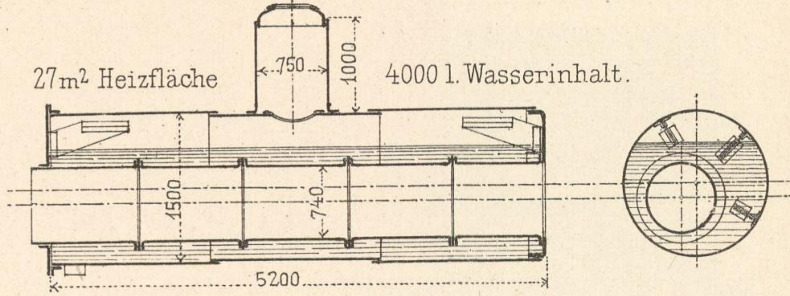
Einflammrohrkessel.
