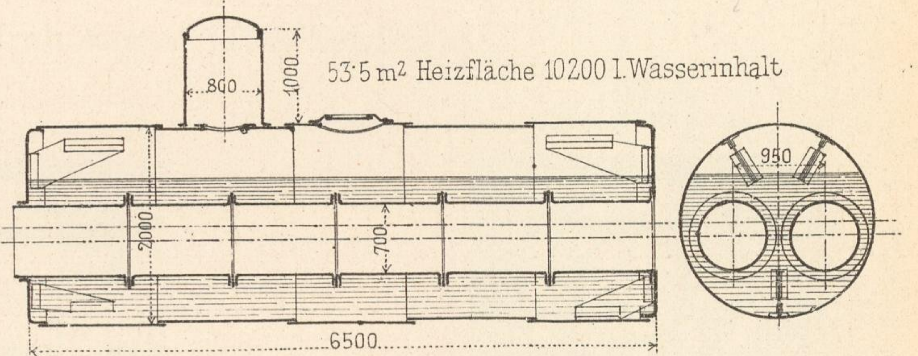
Zweiflammrohrkessel
