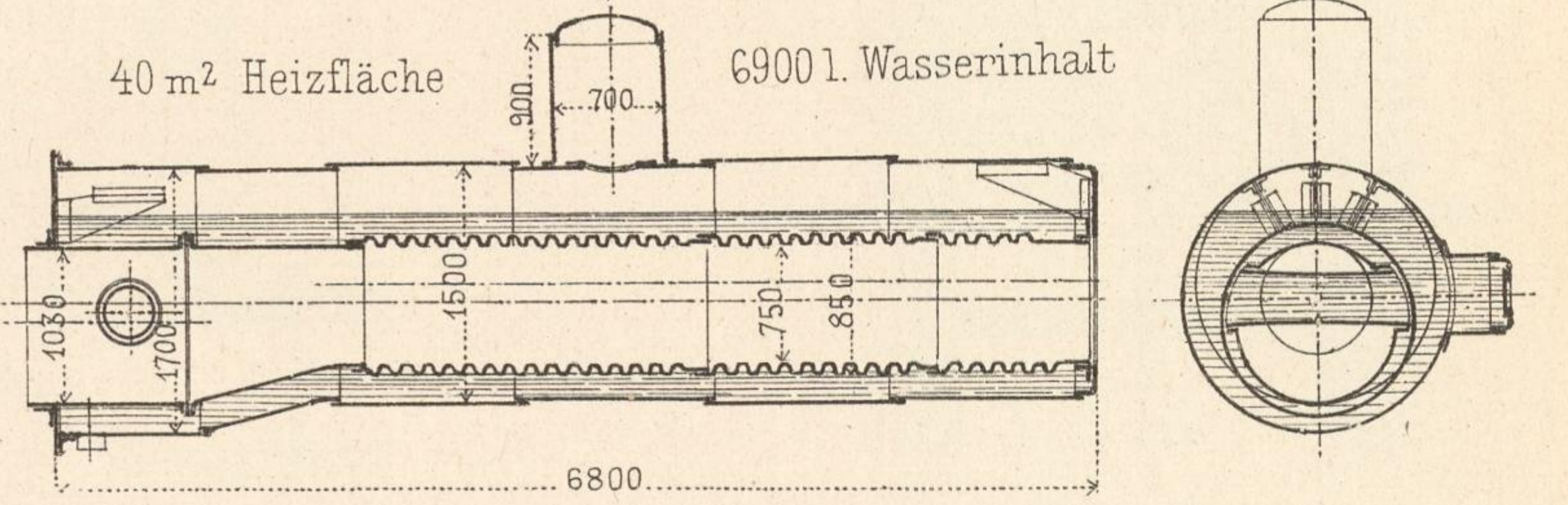
Kuhn'scher Kessel.
