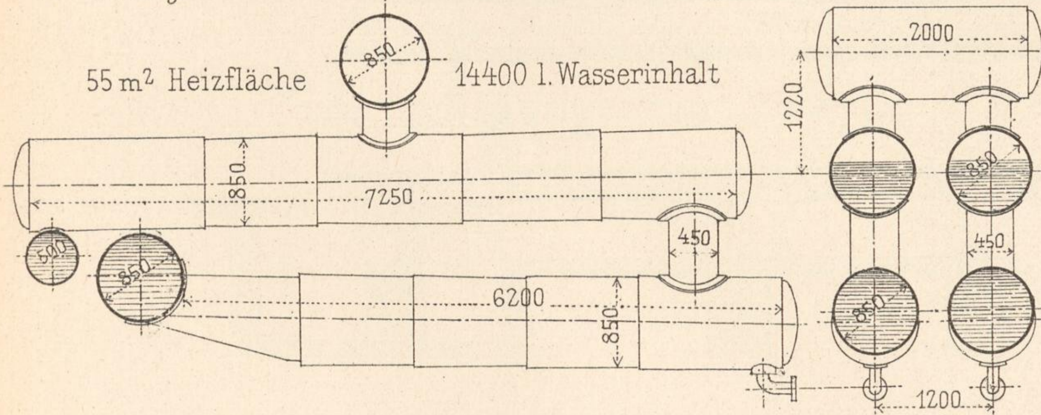
Zweicylinderkessel mit Unterkessel u. Vorlagen.
