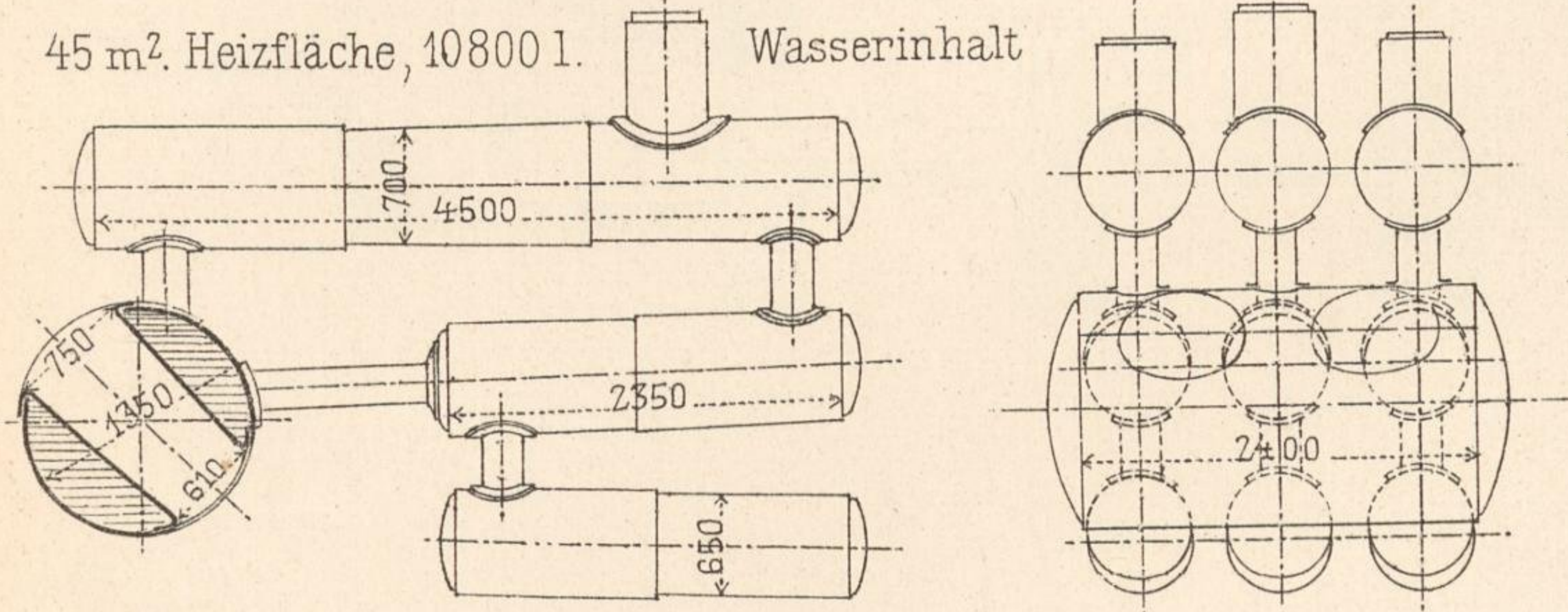
Tenbrinkkessel
