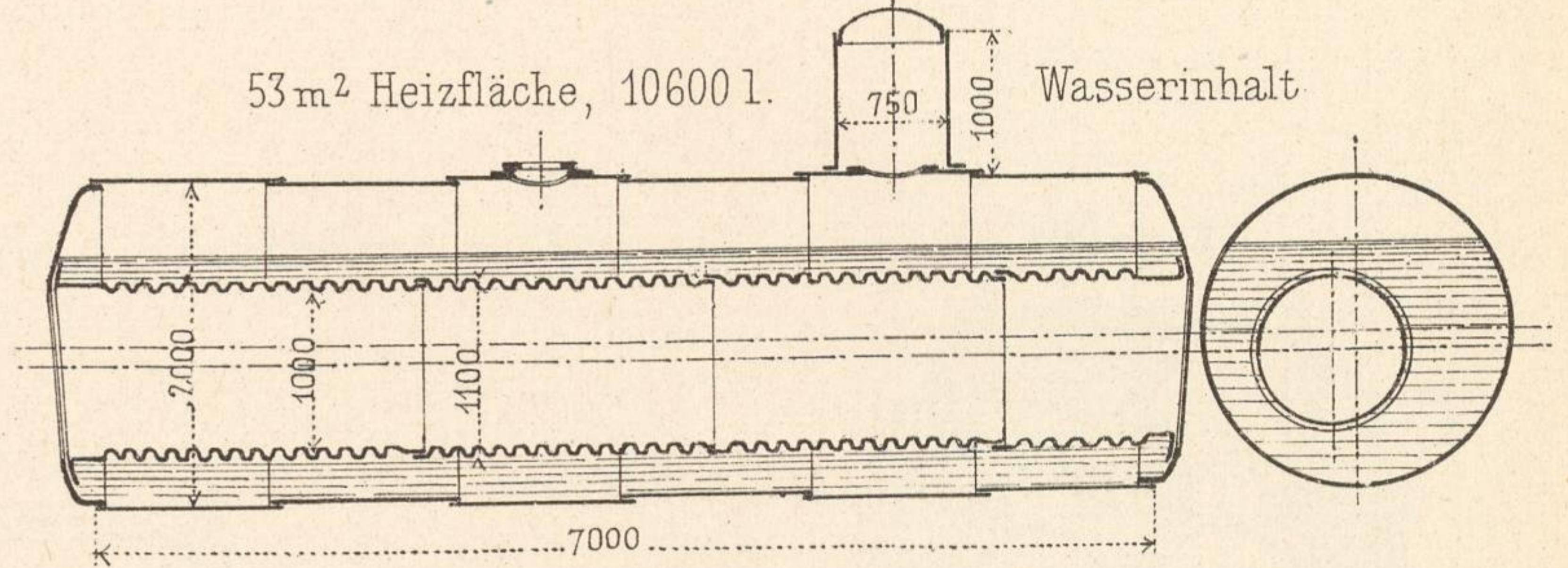
Wellrohrkessel.
