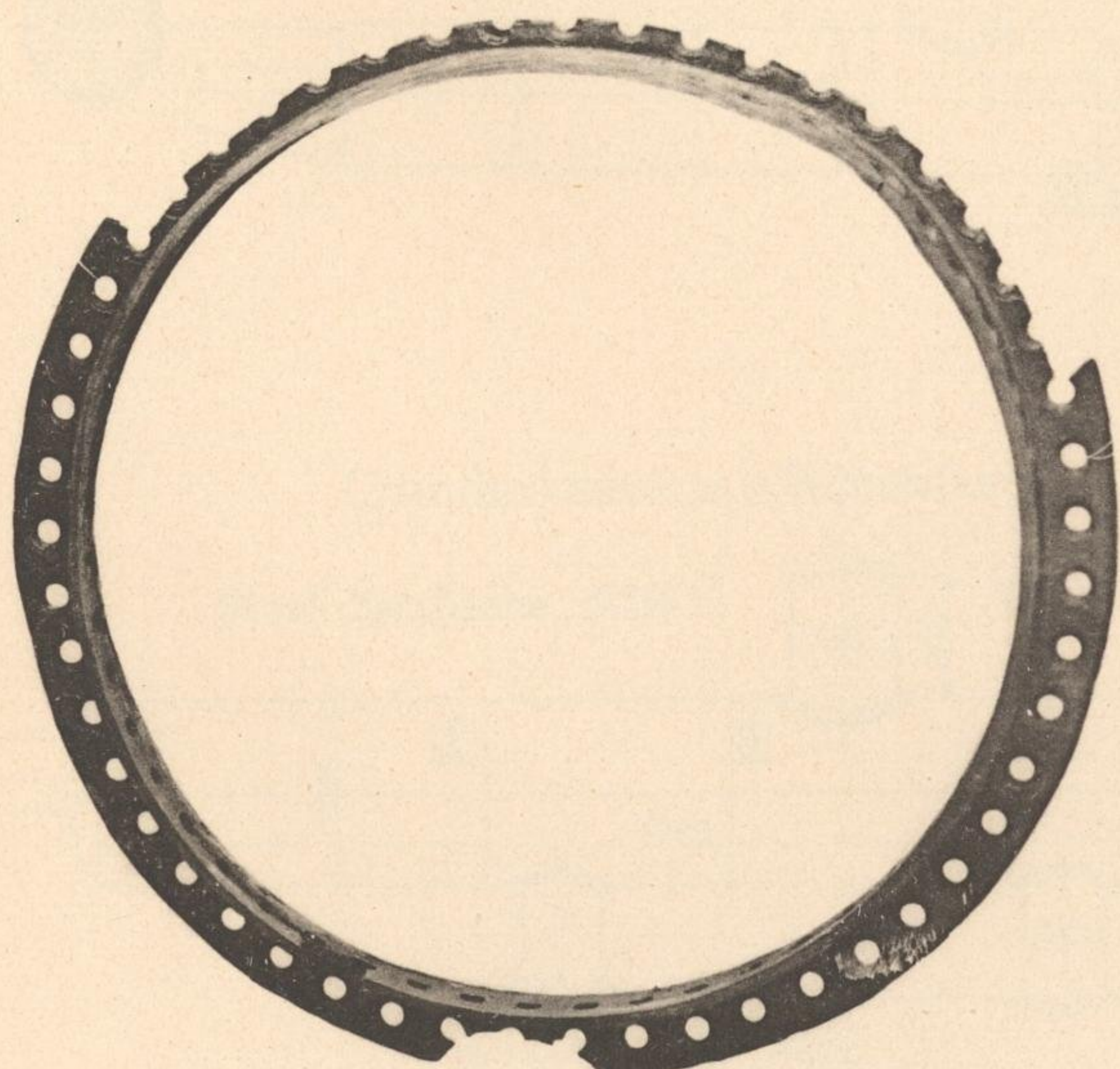
Riss in Winkelringen (27—33).
