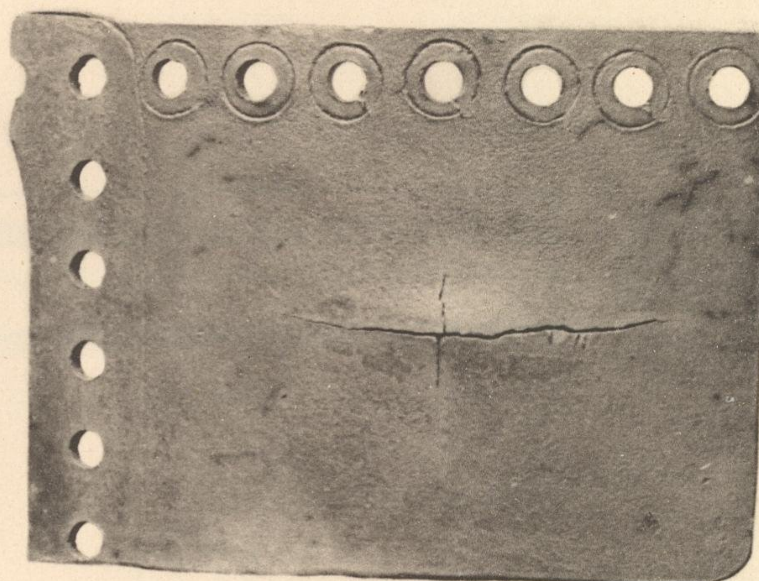
Sternförmiger Riss in der Kesselwand (Aussenseite).
