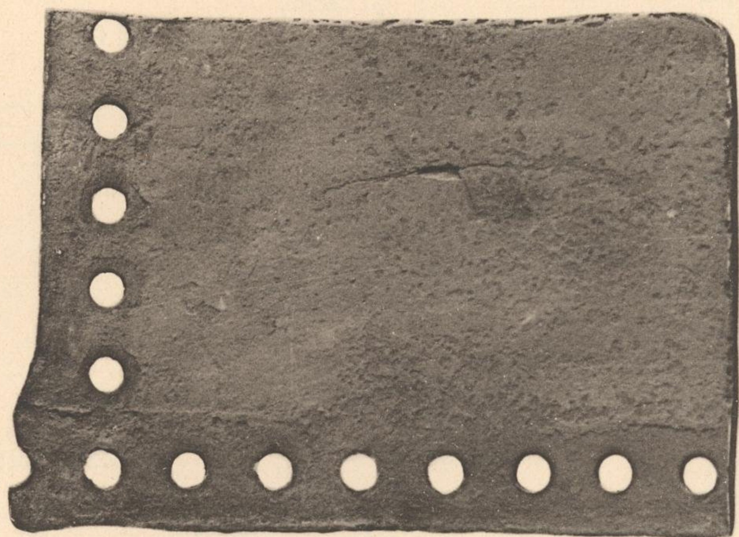
Einfache und verästelte Risse in der Kesselwand (34—36).
