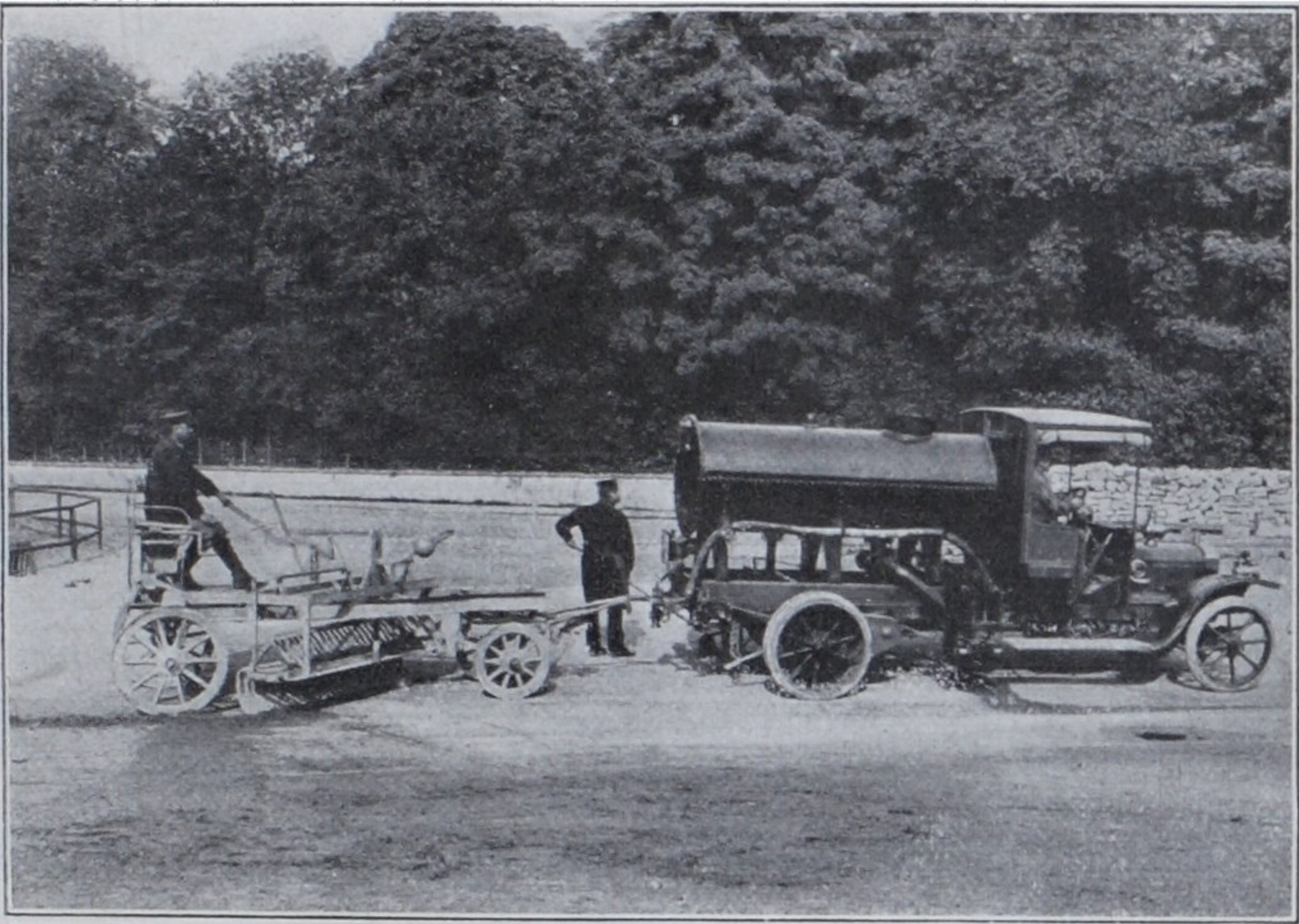
Abb. 46. Fahrbare Krücke.
