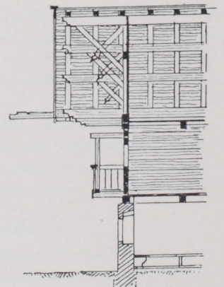
Abb. 2c. Längenschnitt.
