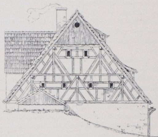
Abb. 23. Ostseite des Hauptgebäudes.
