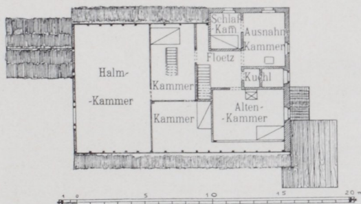
Abb. 24. Dachgeschoß des Hauptgebäudes.
