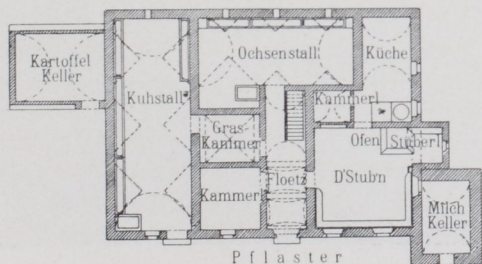
Abb. 25. Erdgeschoß des Hauptgebäudes.
