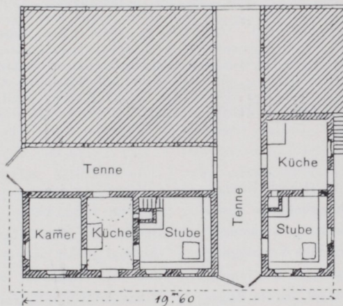
Abb. 2a. Grundriß vom Erdgeschoß.
