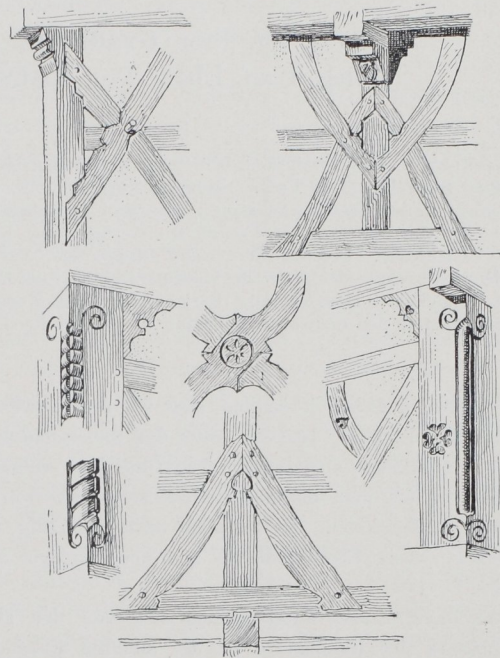
Abb. 59. Fachwerkeinheiten von Blausingen, Kippenheim, Obergrombach, Liedolsheim.
