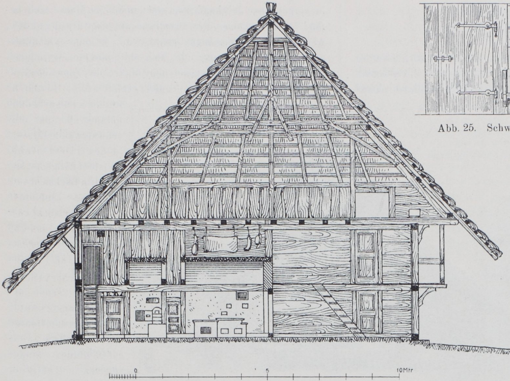
Abb. 22. Querschnitt durch den Wohnhausteil.
