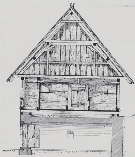
Abb. 16. Querschnitt.
