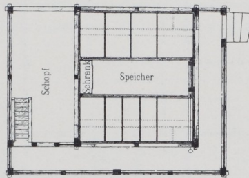
Abb. 13. Obergeschoß.
