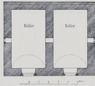
Abb. 14. Kellergeschoß.
