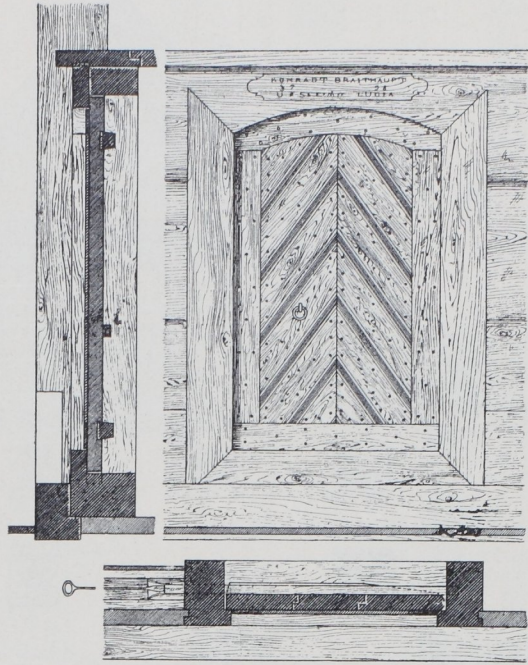
Abb. 17. Speichertüre.
