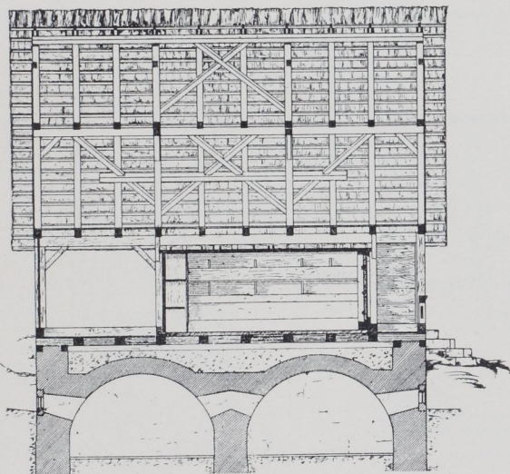
Abb. 15. Längenschnitt.
