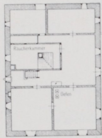
Abb. 53c. Obergeschoß.
